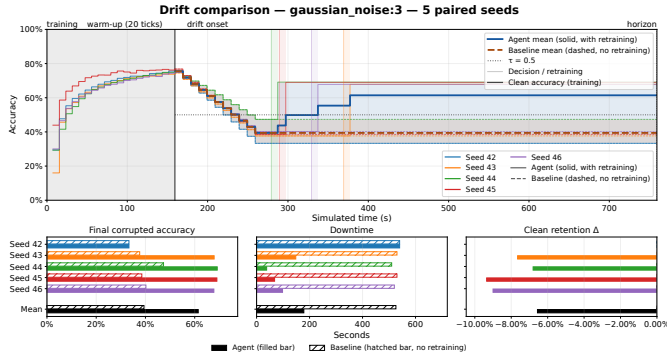
Fig. 3. Ruído Gaussiano, rampa de 100s, cinco seeds pareadas. A seed 42 nunca dispara. Sua trajetória (azul sólida) não se recupera, enquanto as outras quatro seeds se recuperam para cerca de 0,68.
