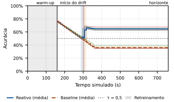
Fig. 2. Motion blur, rampa de 200 s, cinco seeds pareadas. A variante reativa recupera-se em uma rodada e permanece acima de \tau durante a maior parte do horizonte; a baseline segue caindo até cerca de 0,35.
