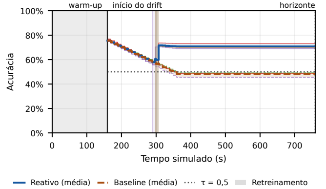
Fig. 1. Fog, rampa de 200 s, cinco seeds pareadas. Acurácia sob degradação ao longo do tempo simulado (sólida: reativo, tracejada: baseline; linhas grossas: médias); \tau = 0,5 tracejada; faixas sombreadas: a rodada de retreinamento. A variante reativa nunca cai abaixo de \tau (downtime zero).
