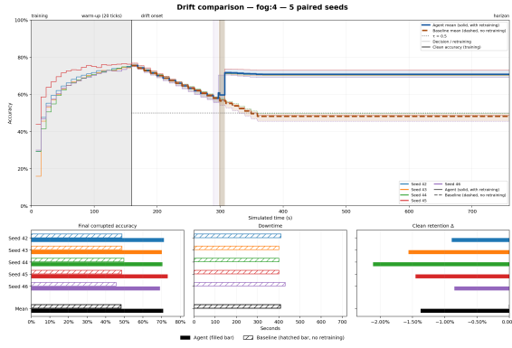
Fig. 1. Névoa, rampa de 200s, cinco seeds pareadas. Acima: acurácia corrompida ao longo do tempo simulado (sólida: reativo, tracejada: linha de base; linhas grossas: médias); \tau = 0,5 tracejada; faixas sombreadas: a rodada de retreinamento. Abaixo: acurácia final corrompida, indisponibilidade e retenção limpa; o braço reativo nunca cai abaixo de \tau (indisponibilidade zero).
