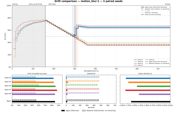
Fig. 2. Motion blur, rampa de 200s, cinco seeds pareadas. O braço reativo recupera-se em uma rodada e permanece acima de \tau durante a maior parte do horizonte; a baseline segue caindo até cerca de 0,35.
