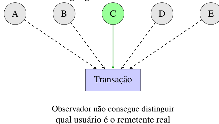
Figura 10 – Funcionamento das Ring Signatures
