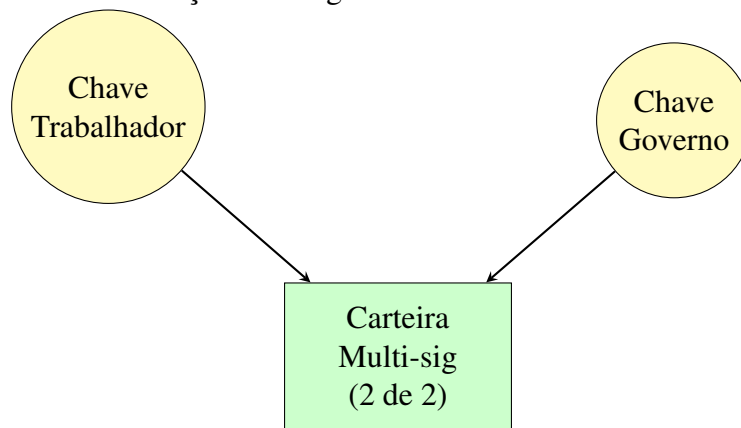
Figura 7 – Sistema de Governança Multi-sig
