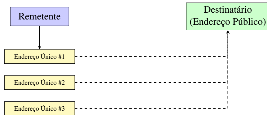
Figura 11 – Funcionamento dos Stealth Addresses
