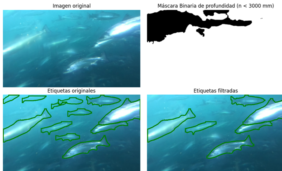
Figura 12.16: Implementación del filtro de profundiad. Como puede verse en la máscara binaria de la derecha, algunas instancias se encuentran fuera del umbral de distancia (en este caso 3 metros) y por ende son excluidos del dataset .
