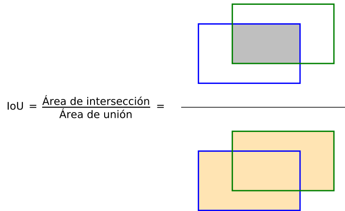
Figura 7.14: Intersección sobre la unión.
