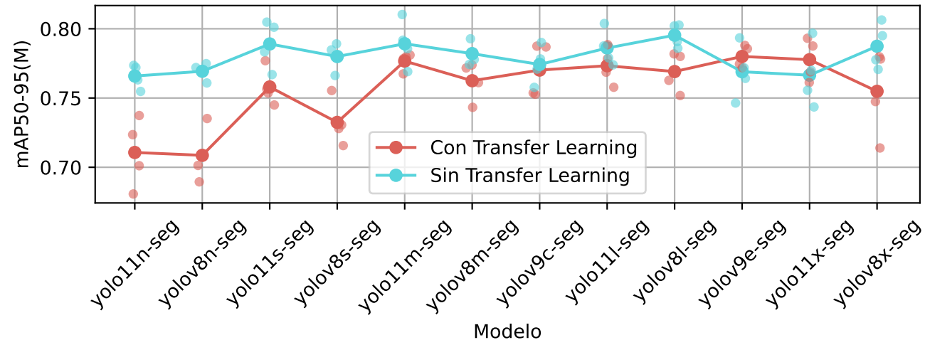
Resultados con exportación TensorRT-INT8
