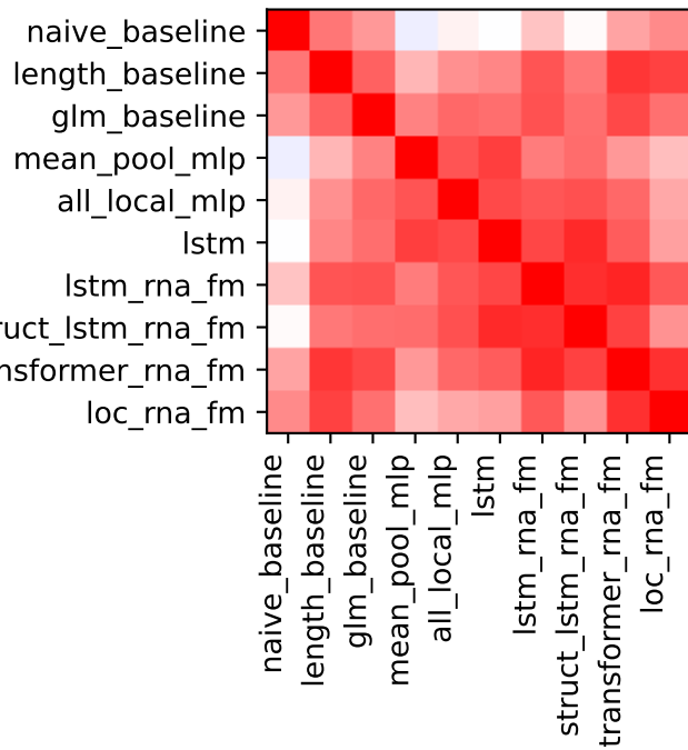
KL Divergence
