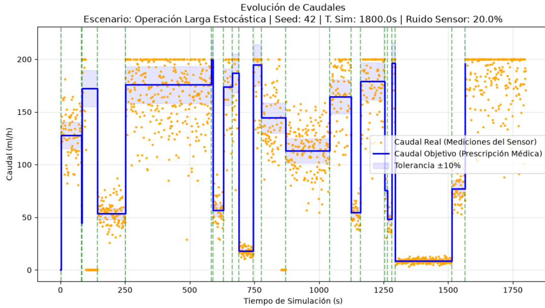
Figura 4.1: Evolución temporal del caudal de la bomba. Se compara el caudal objetivo prescrito y el caudal real basado en las mediciones del sensor. La franja sombreada representa el margen de tolerancia operativa del \pm 10\% . Las líneas verticales verdes indican el ingreso de nuevas órdenes médicas.
