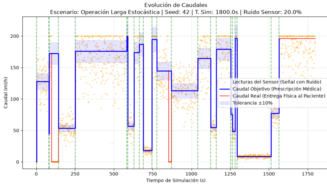
Figura 4.1: Evolución temporal del caudal de la bomba. Se compara el caudal objetivo prescrito, el caudal real entregado al paciente y las lecturas ruidosas individuales del sensor. La franja sombreada representa el margen de tolerancia operativa del \pm 10\% . Las líneas verticales verdes indican el ingreso de nuevas órdenes médicas.
