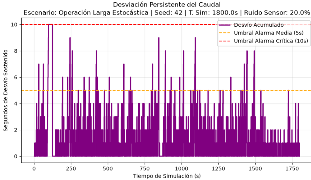
Figura 4.2: Acumulación de segundos de desviación sostenida respecto a los umbrales lógicos del sistema. La caída abrupta a cero indica que el caudal retornó a la normalidad.
