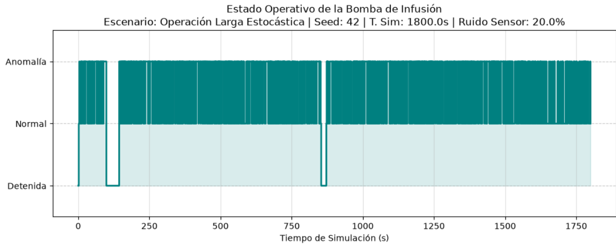
Figura 4.4: Diagrama de transiciones de estado de la bomba de infusión. Permite identificar de un vistazo las ventanas de detención, operación segura y los períodos de anomalía.
