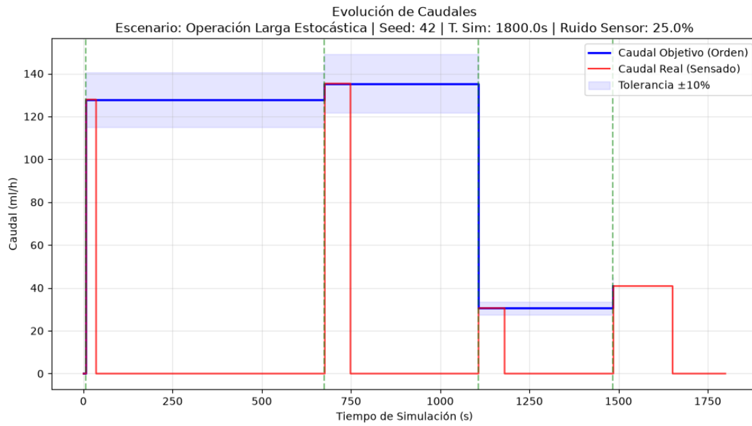
Figura 4.1: Evolución temporal del caudal objetivo versus el caudal sensado por el dispositivo. La franja sombreada representa el margen de tolerancia operativa del \pm 10\% . Las líneas verticales verdes indican el ingreso de nuevas órdenes médicas.
