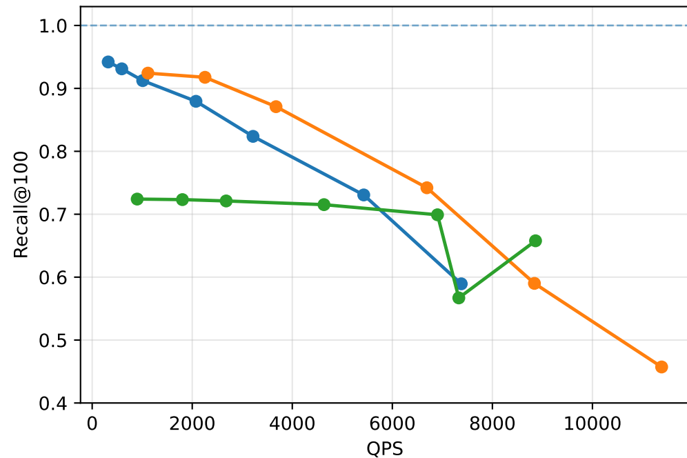
MiniLM
