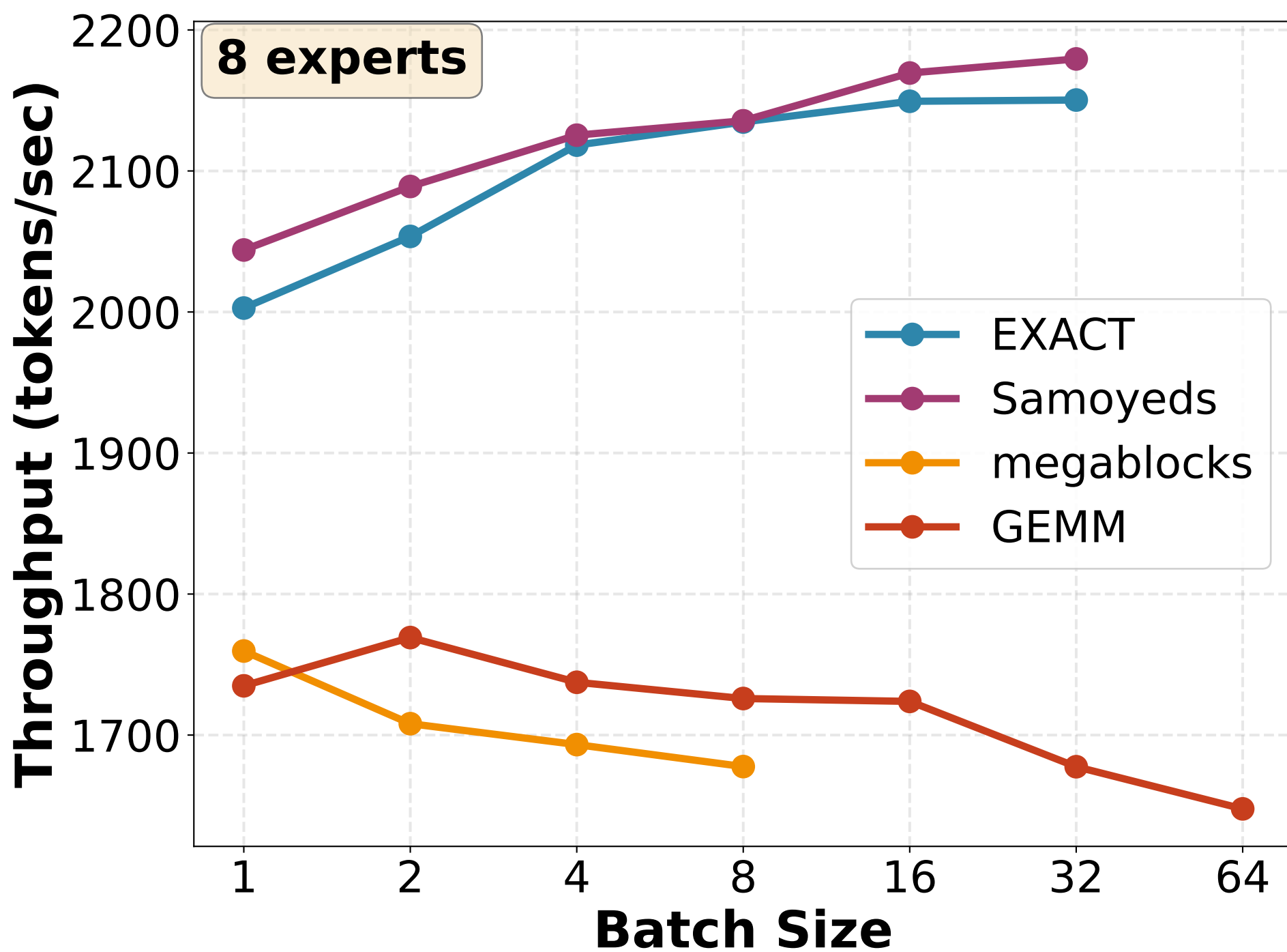
DeepSeek-MoE-16B
