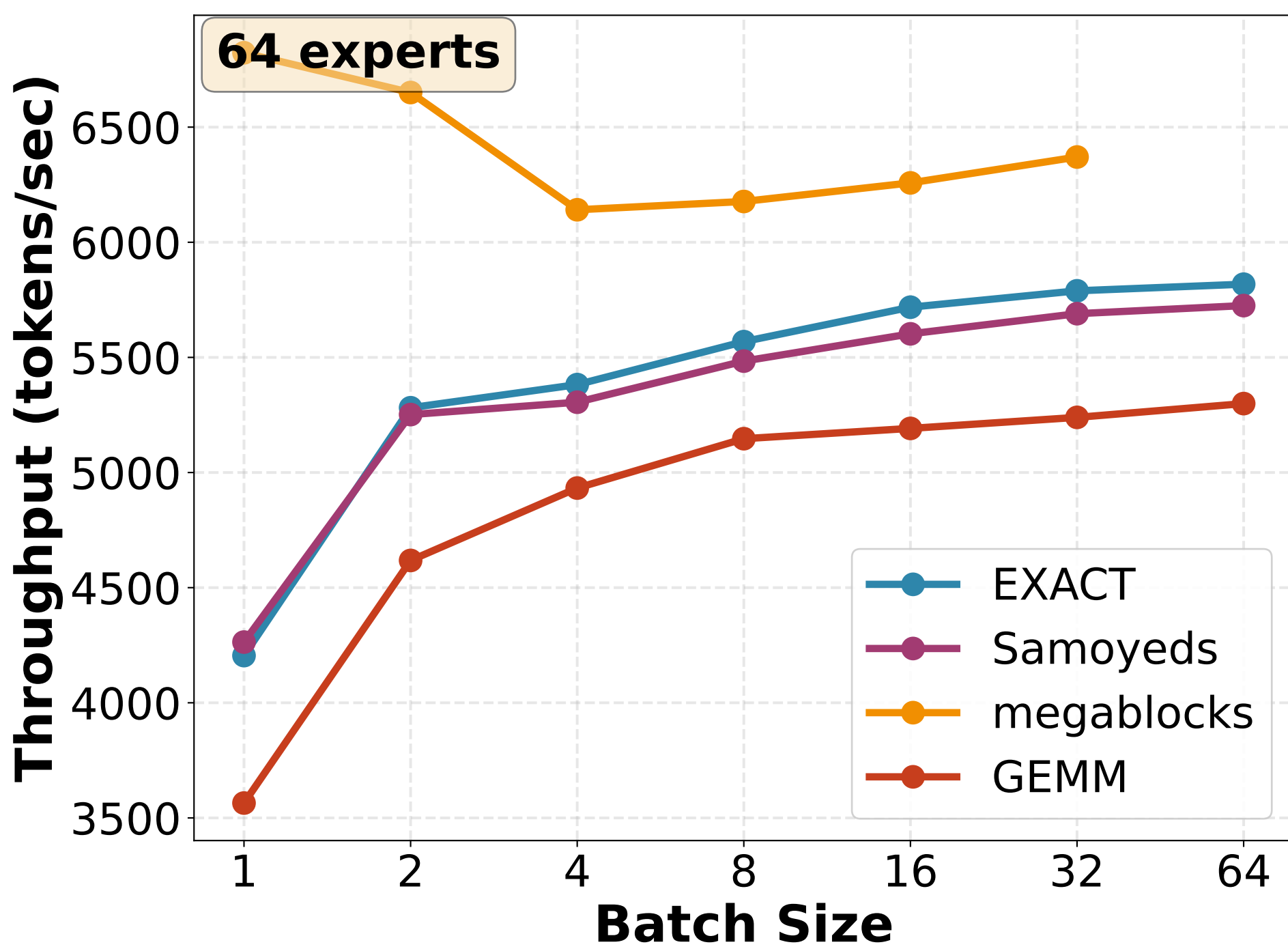
DeepSeek-MoE-16B
