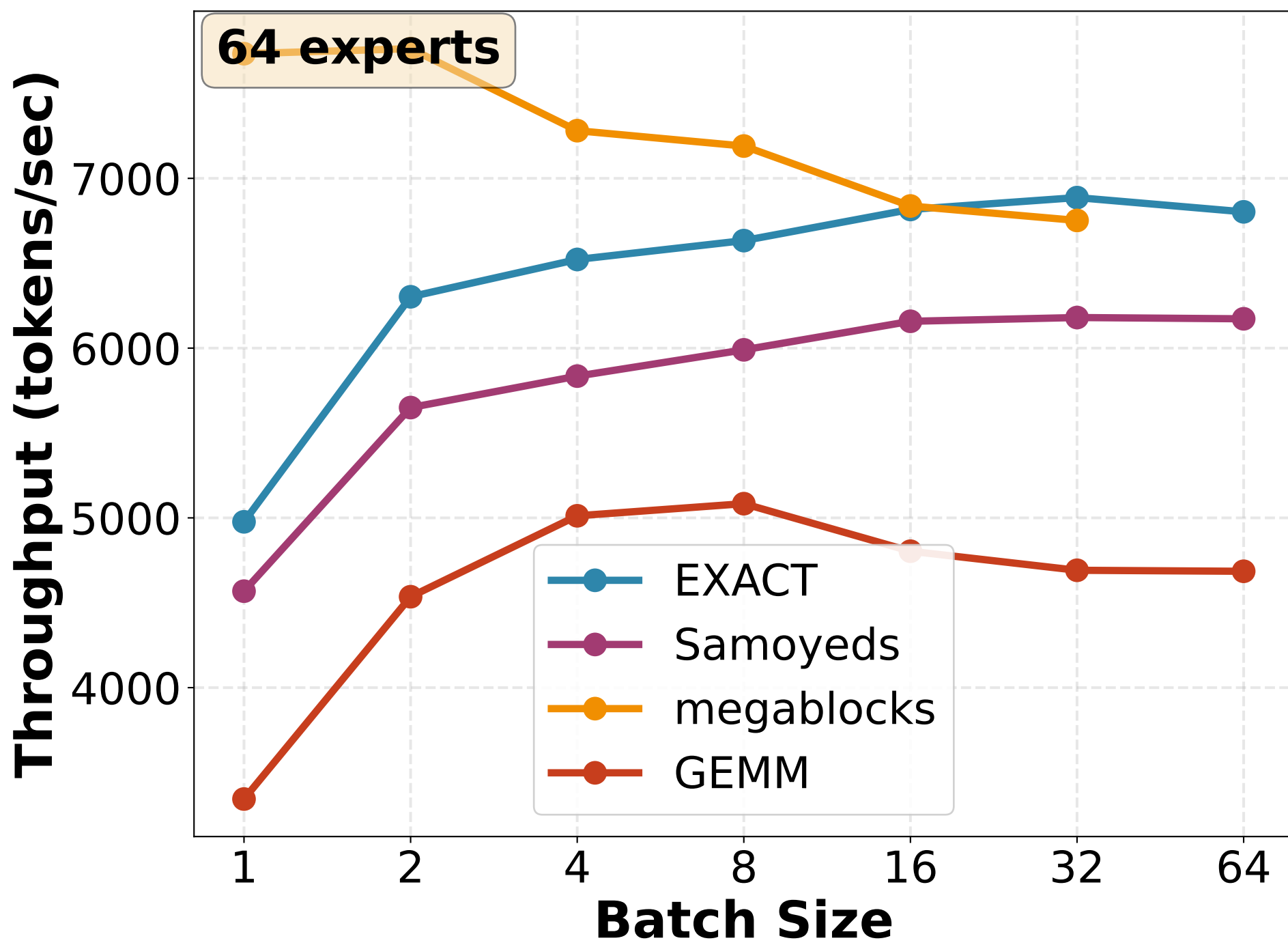
DeepSeek-MoE-16B
