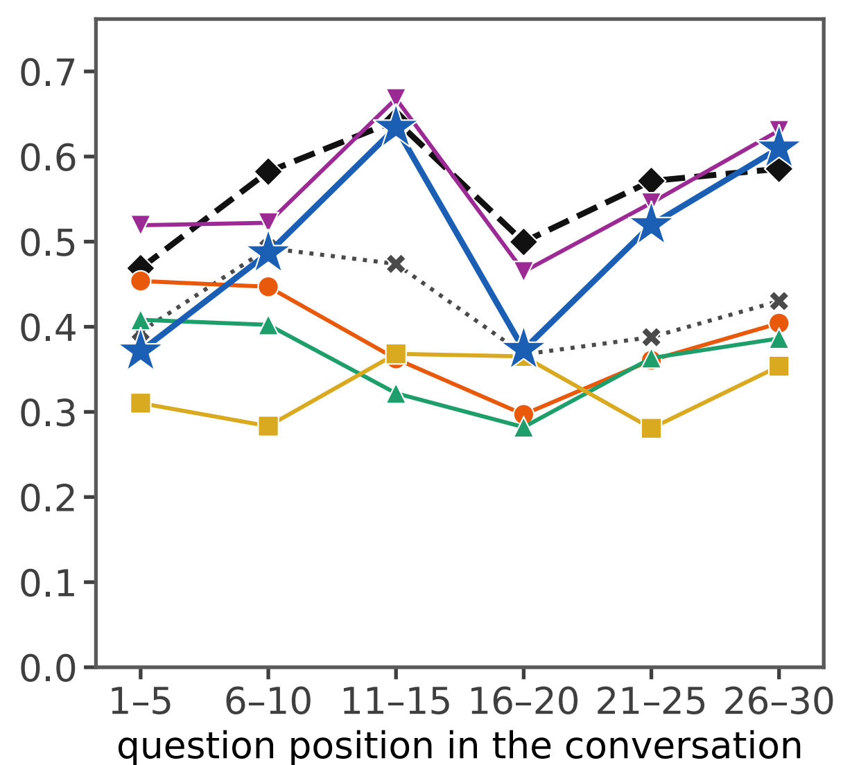
(b) LoCoMo
