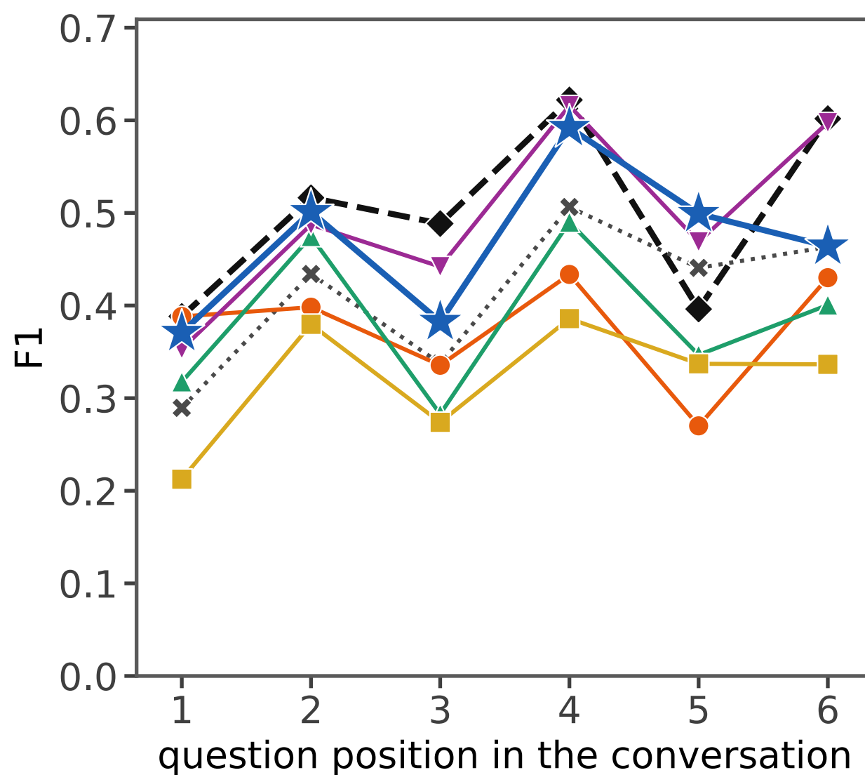
(a) LooGLE
