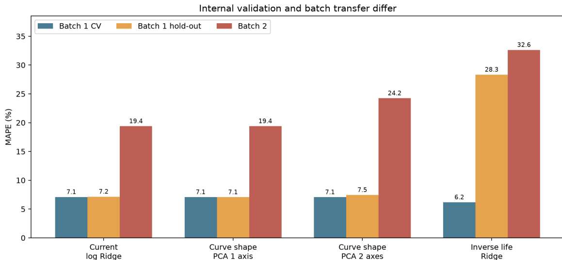
새 접근의 정책별 CV, hold-out, Batch 2 MAPE 비교
