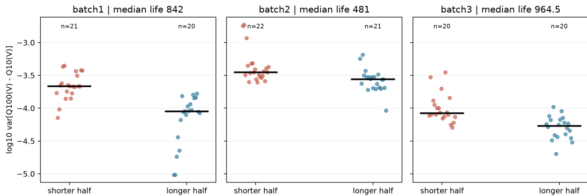
배치별 수명 중앙값으로 나눈 두 집단의 \Delta Q(V) 로그 분산: 점은 셀, 검은 선은 중앙값
