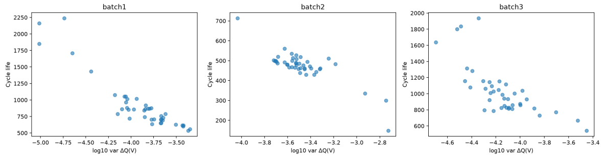
\Delta Q(V) 로그 분산과 수명
