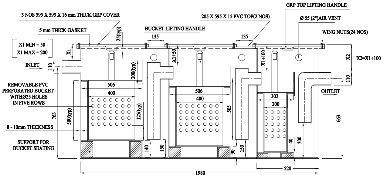
SEC A-A
