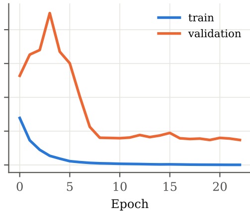
CNN-BiLSTM
