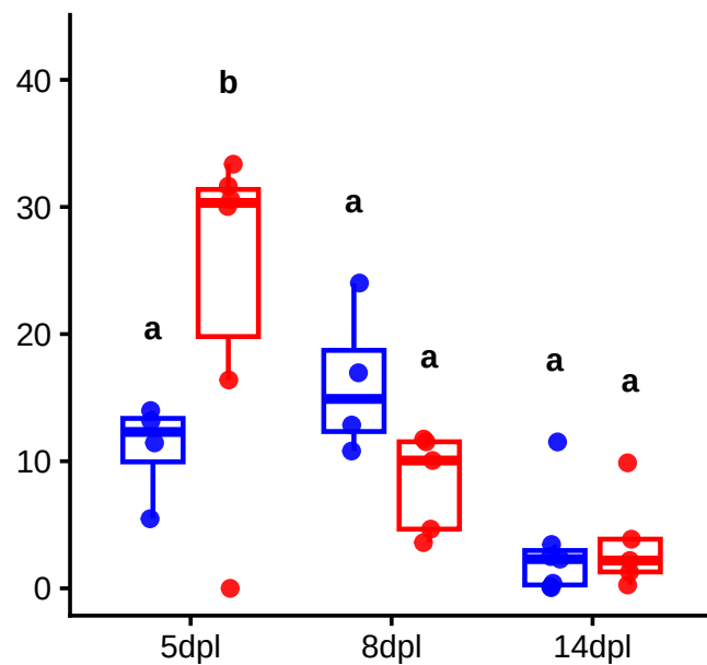
Caspase – Inoc
