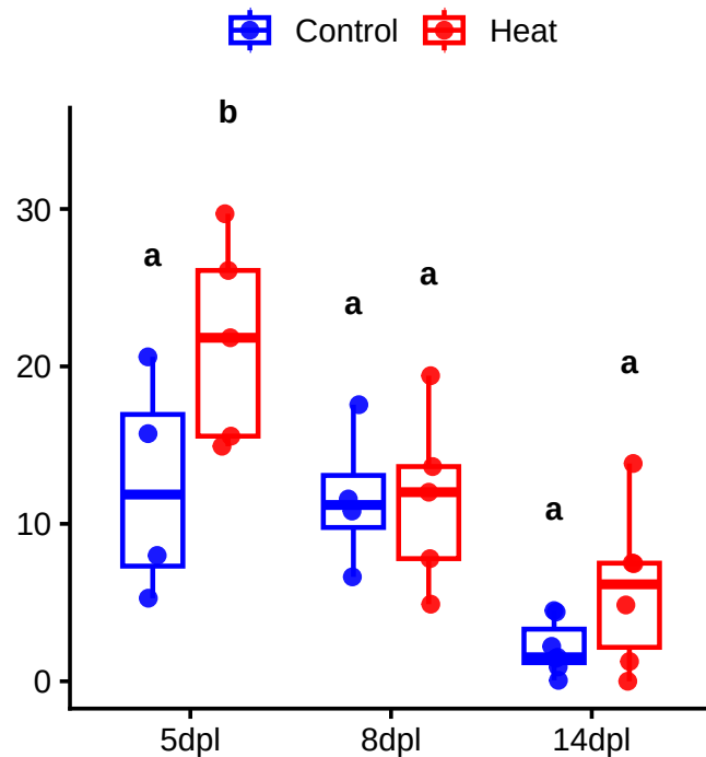
Caspase – Inoc
