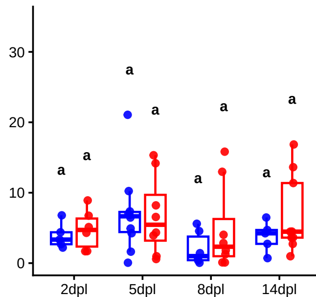
Caspase – Sym
