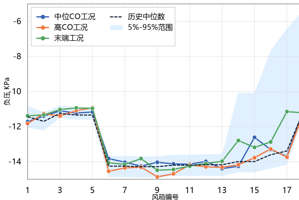
图 3 典型工况推荐负压曲线
