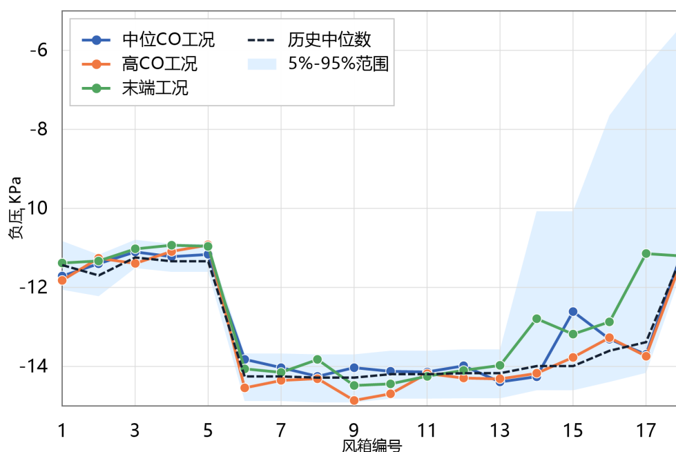
图 4 典型工况推荐负压曲线
