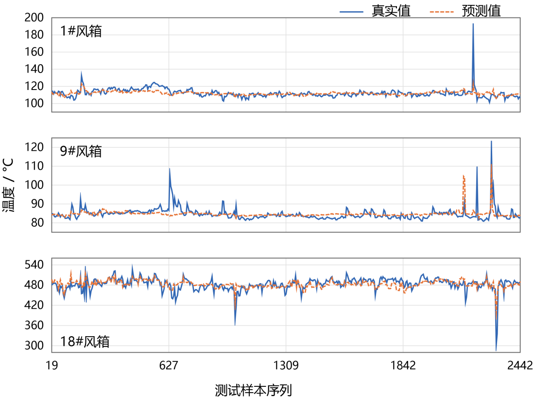
图 3 代表风箱温度预测效果
