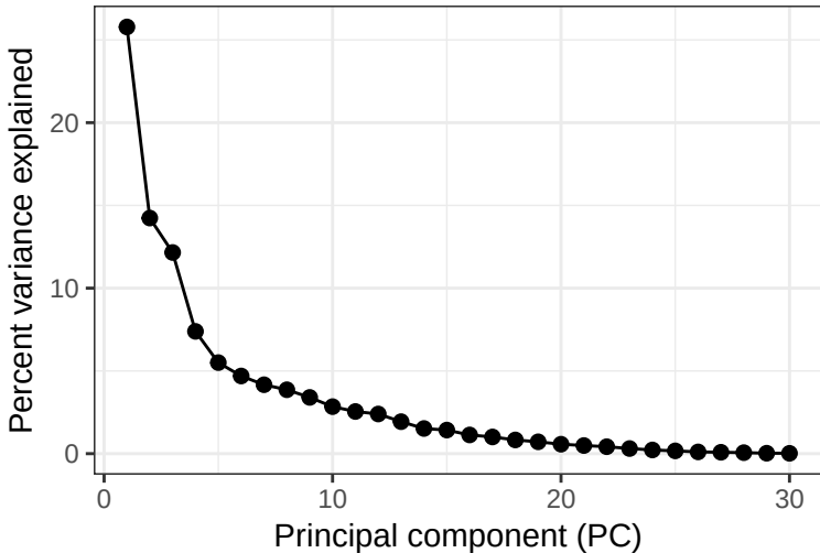
PCA elbow plot
