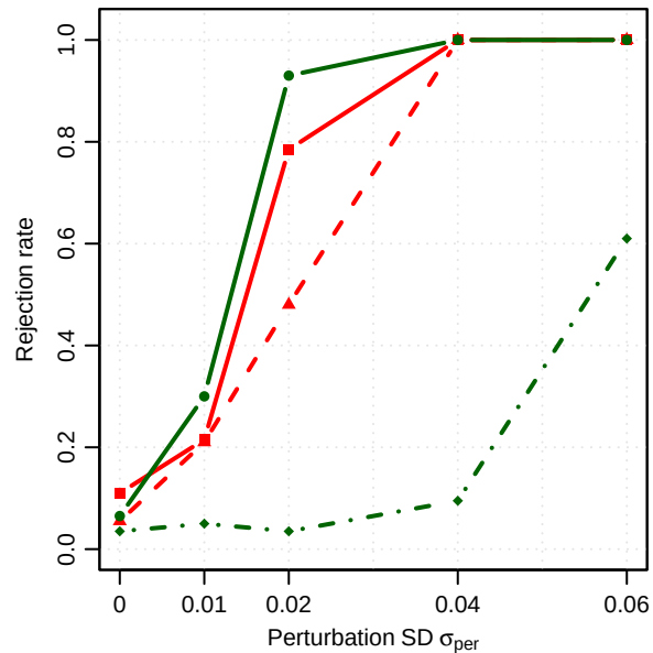
(b) RBM, perturb all B
