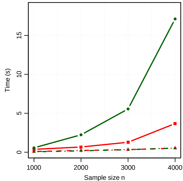
(d) Runtime (RBM)
