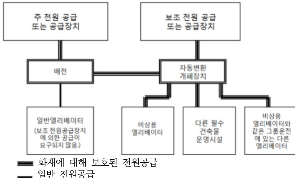
[ 그림 29 - 소방구조용 엘리베이터의 전원공급에 대한 예시 ]
