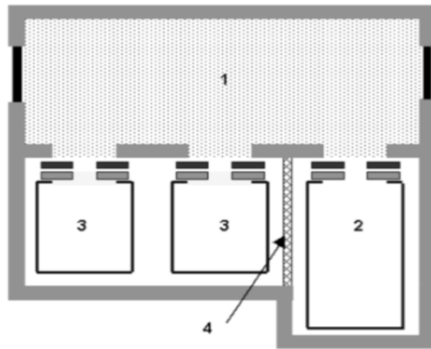
[ 그림 24.2 - 다수의 승강로에 있는 소방구조용 엘리베이터 및 방화 구획된 로비의 배치도 ]
