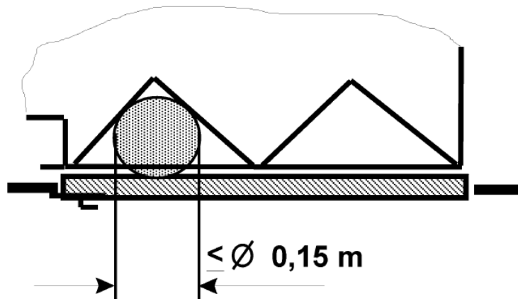
[ 그림 6 - 경첩달린 승강장문과 접힌 카문의 틈새 ]
