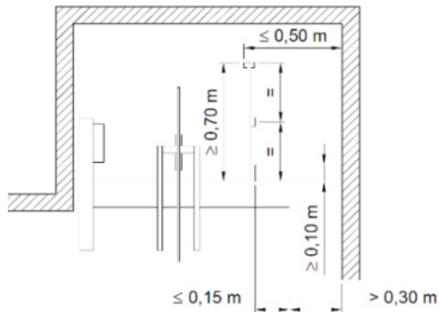
〈 0.7 m 이상의 보호난간 필요, 발보호판 높이 0.1 m 이상 〉
