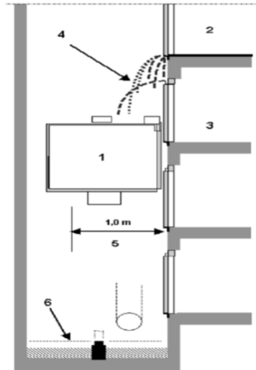
[ 그림 26 - 전기장치의 물에 대한 보호 ]
