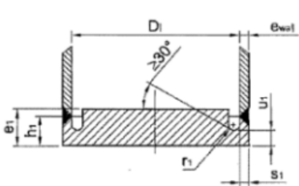
[ 그림 XI.2 - 릴리빙 홈을 가진 평평한 기초 ]
