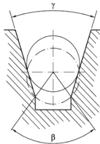
[ 그림 IX.2 V-홈 ]
