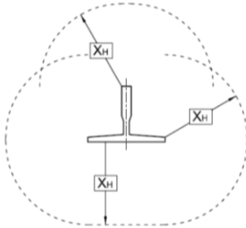
[ 그림 6. 주행안내 레일 주변의 수평 거리 X_H ]
