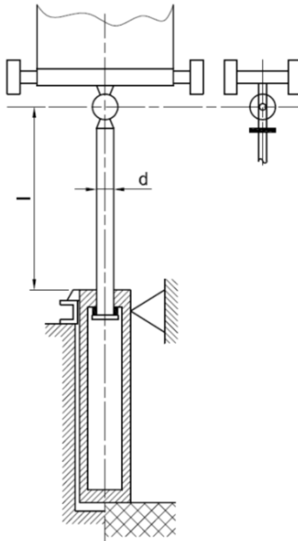
[ 그림 XI.5 - 단 작동 잭 ]
