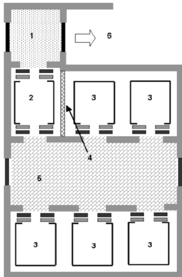
[ 그림 24.3 - 다수의 승강로에 있는 이중 출입 소방구조용 엘리베이터 및 방화 구획된 로비의 배치도 ]
