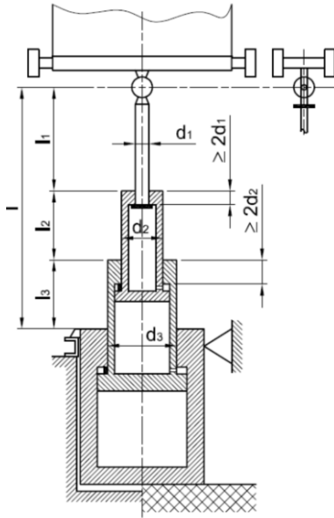
[ 그림 XI.6 - 외부 안내 없는 다단 잭 ]
