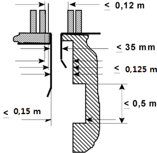
[ 그림 5 - 카와 카 출입구를 마주하는 벽 사이의 틈새 ]
