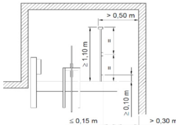
〈 1.1 m 이상의 보호난간 필요, 발보호판 높이 0.1 m 이상 〉
