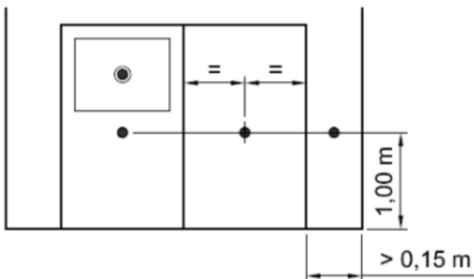
〈사. 문짝과 측면 문틀로 구성된 완전한 승강장 도어 (가 및 나에 따른 예시)〉
