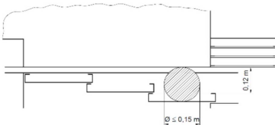
[ 그림 10. 기계적으로 연동되지 않은 수평 개폐식 승강장문과 카문의 조합 ]
