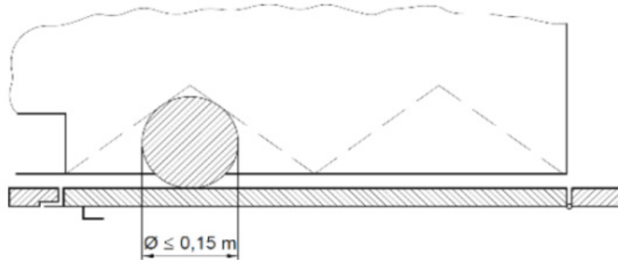
[ 그림 8. 경첩이 있는 승강장문과 접히는 카문의 조합 ]
