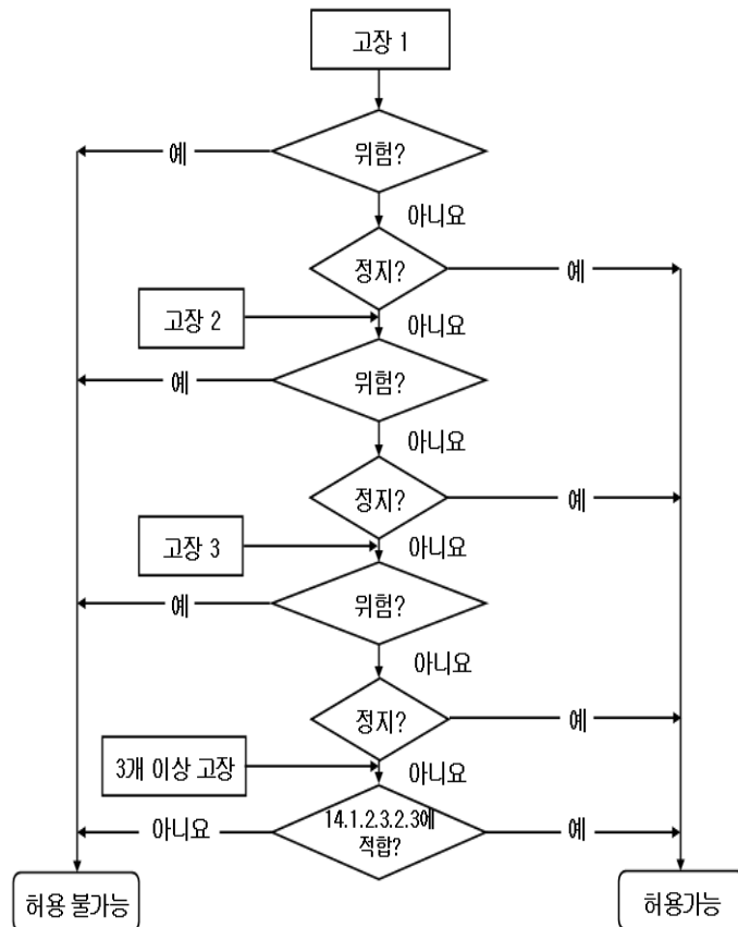
[ 그림 7 안전회로 평가 도표 ]
