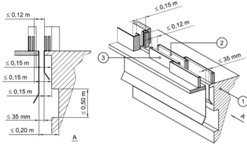
[ 그림 3. 카와 카 출입구를 마주하는 벽 사이의 틈새 ]
