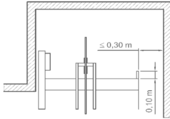
〈 보호난간 불필요, 발보호판 높이 0.1 m 이상 〉
