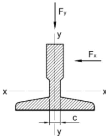
[ 그림 Ⅷ.1 - 주행안내 레일의 축 ]
