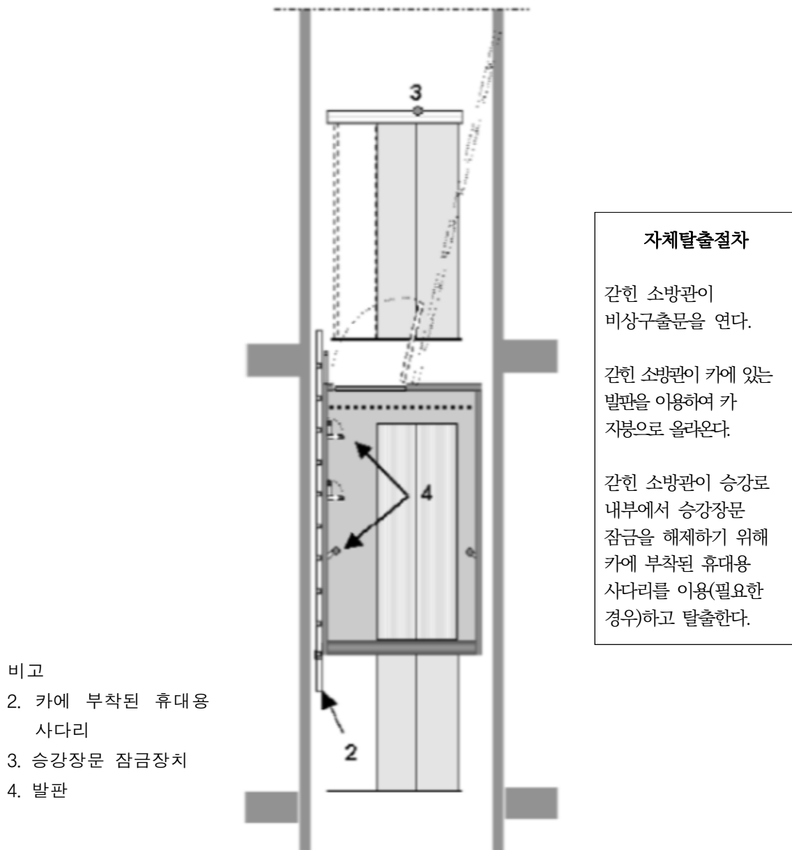
[ 그림 27.2 - 카에 부착된 휴대용 사다리를 이용한 자체 탈출 ]
