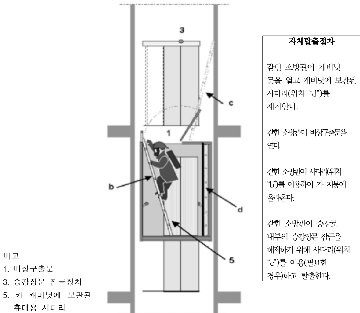
[ 그림 27.3 - 카 내부 캐비닛에 보관된 휴대용 사다리를 이용한 자체 탈출 ]
