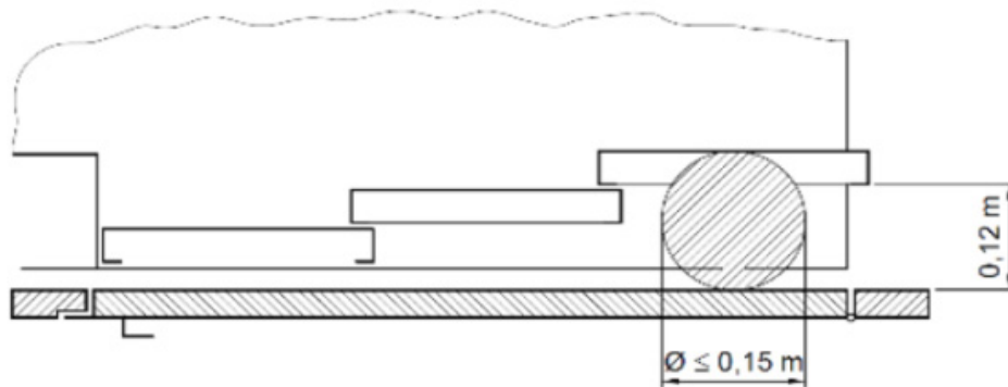
[ 그림 9. 경첩이 있는 승강장문과 수평 개폐식 카문의 조합 ]
