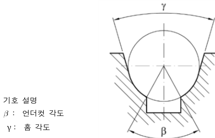
[ 그림 IX.1 반원 언더컷 홈 ]
