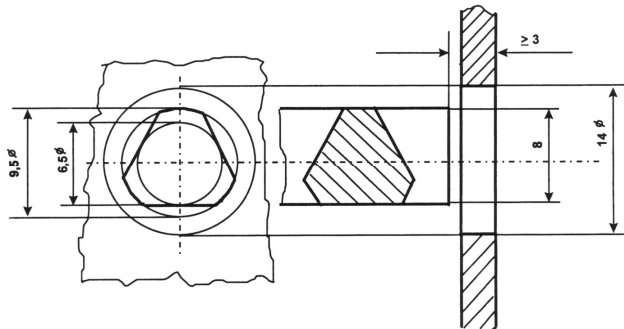
〈그림 3〉 열쇠구멍(unlocking triangle)
