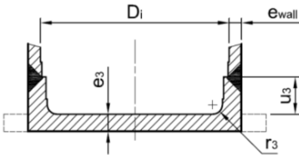
[ 그림 XI.4 - 플랜지 용접된 편평한 기초 ]
