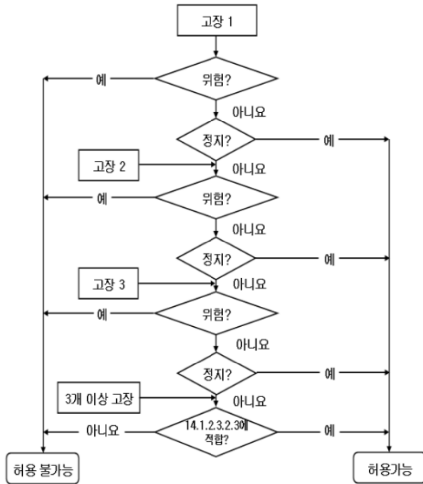
[ 그림 21 - 안전 회로 평가를 위한 순서도 ]
