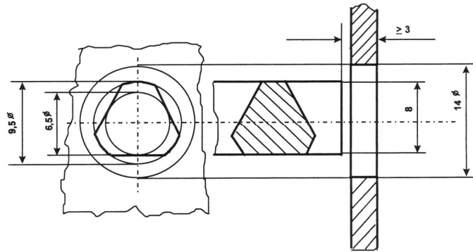
〈그림 3〉 열쇠구멍(unlocking triangle)
