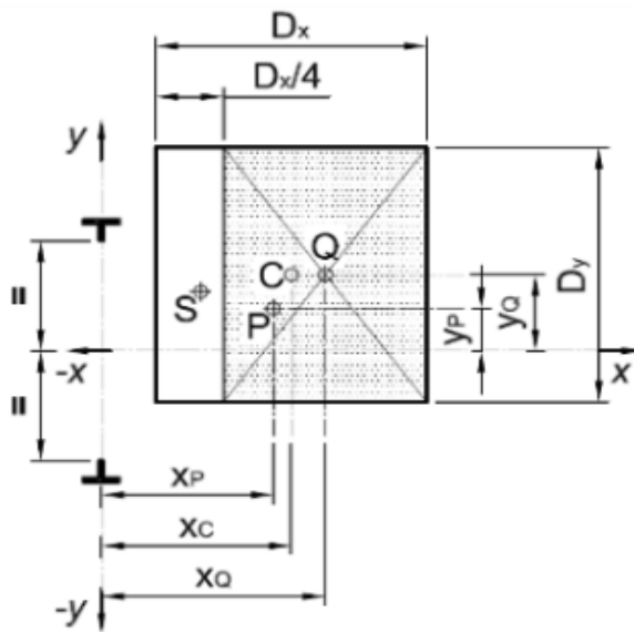
[ 그림 VIII.4 - 추락방지안전장치 작동 - 엘리베이터 카의 하중 분포(X-축에 대해) ]
