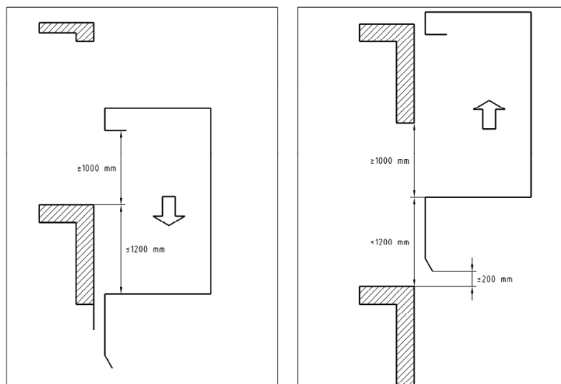
[ 그림 4 의도되지 않은 카의 움직임 ]
