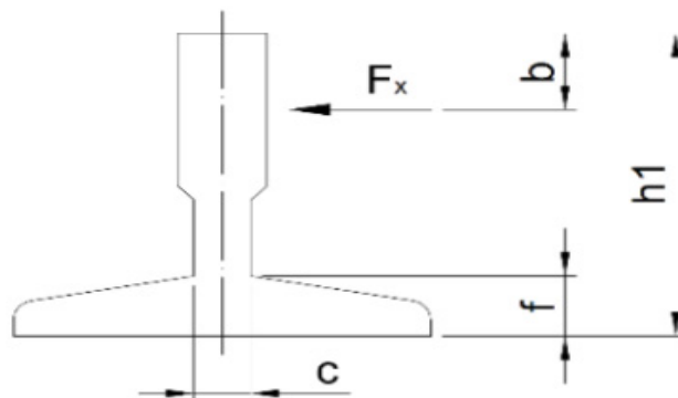
[ 그림 VIII.2 - 플랜지 굽힘 계산의 치수 ]
