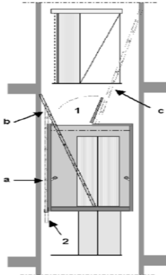
[ 그림 27.1 - 카에 부착된 휴대용 사다리를 이용하여 승강로 밖으로 구출 ]
