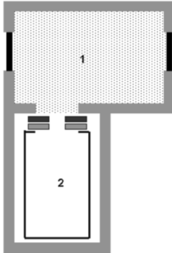
[ 그림 24.1 - 단독 소방구조용 엘리베이터 및 방화 구획된 로비의 배치도 ]
