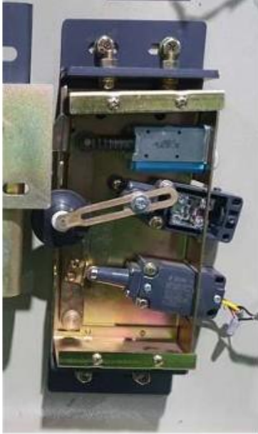
전자식 인터록 예시 (일명: 전자인터록)
