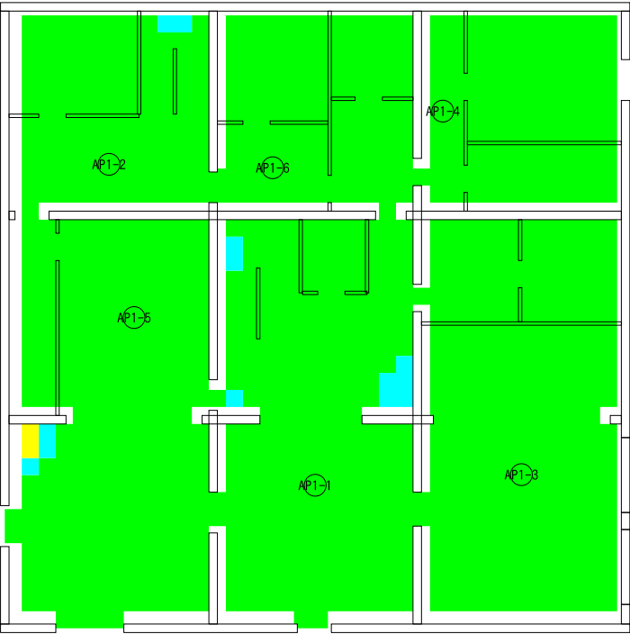
1階（AP 6台・目標を満たす面積 100%）
