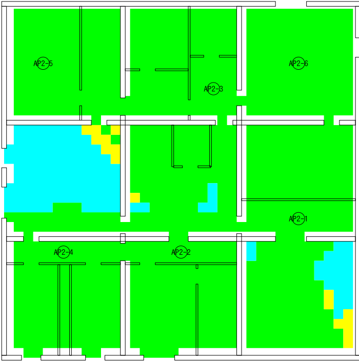
2階（AP 6台・目標を満たす面積 99%）
