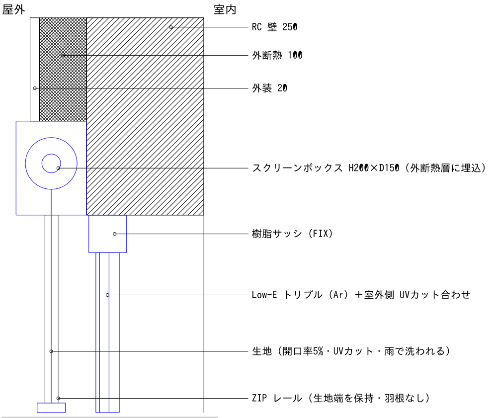
(5) 窓上部 断面詳細（模式図 1:8）
