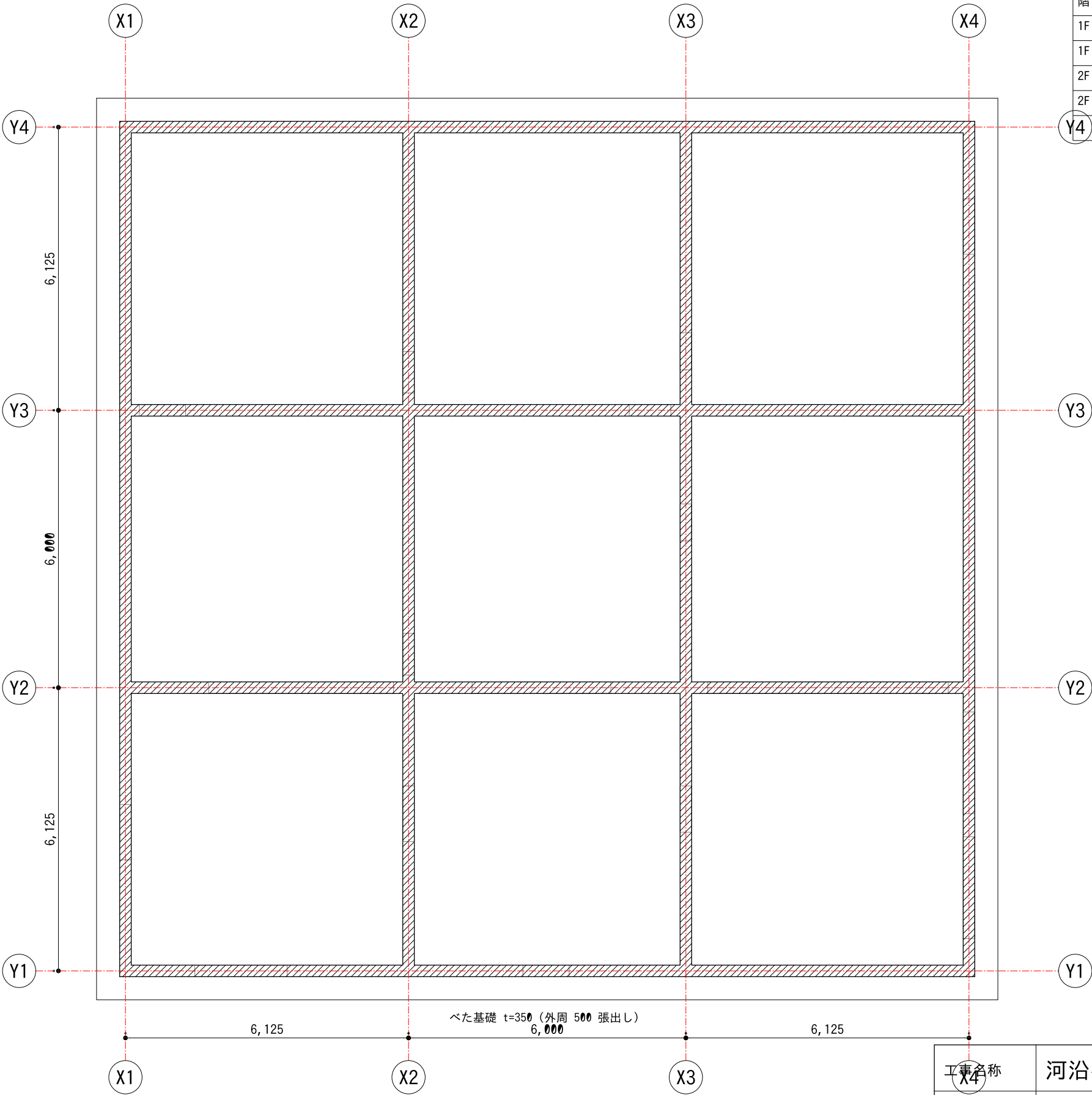
基礎伏図・耐力壁配置図（1階） S=1:100 網掛け=RC耐力壁 t=250（1・2階 同位置）、破線=開口
