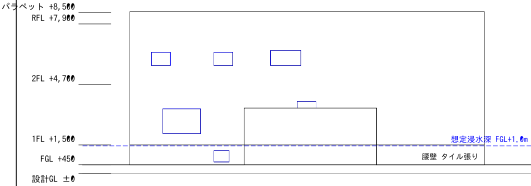
南立面図
