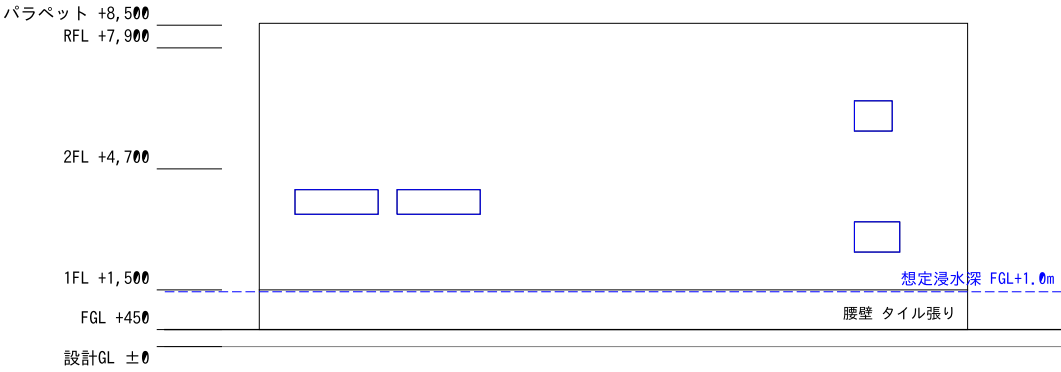
東立面図
