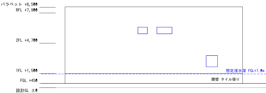
西立面図
