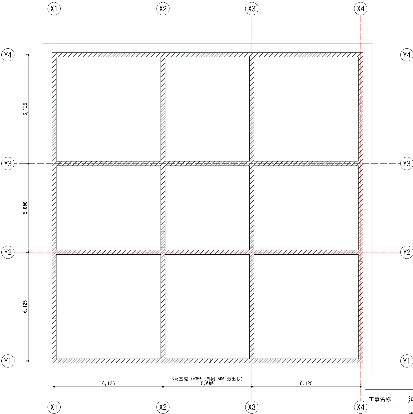
基礎伏図・耐力壁配置図（1階） S=1:100
