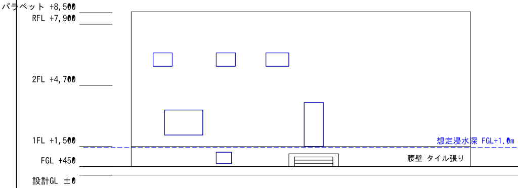
南立面図
