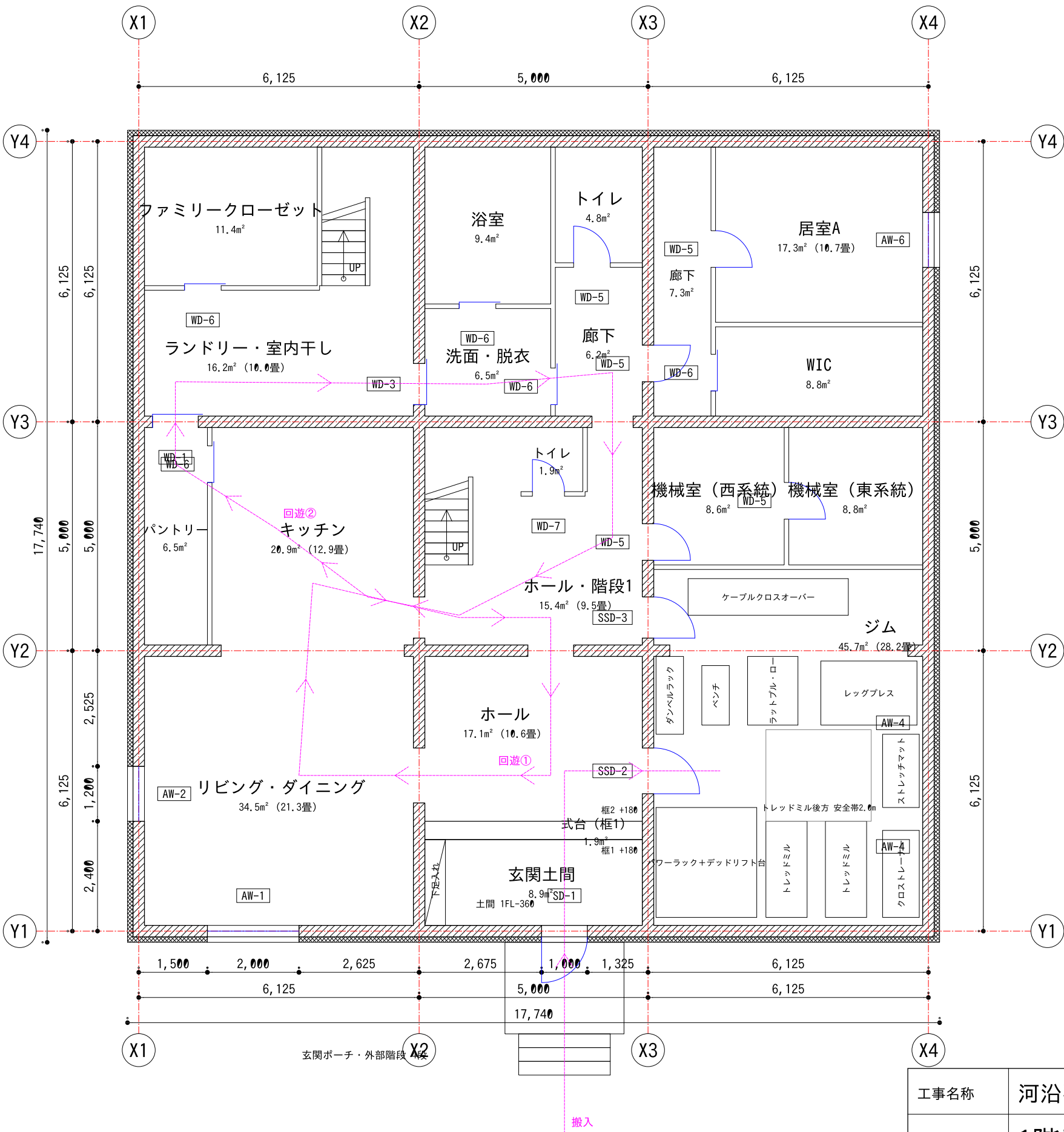
1階平面図 S=1:100 1FL = 設計GL+1,500 (TP+110.50) / 天井高 CH=2,600
