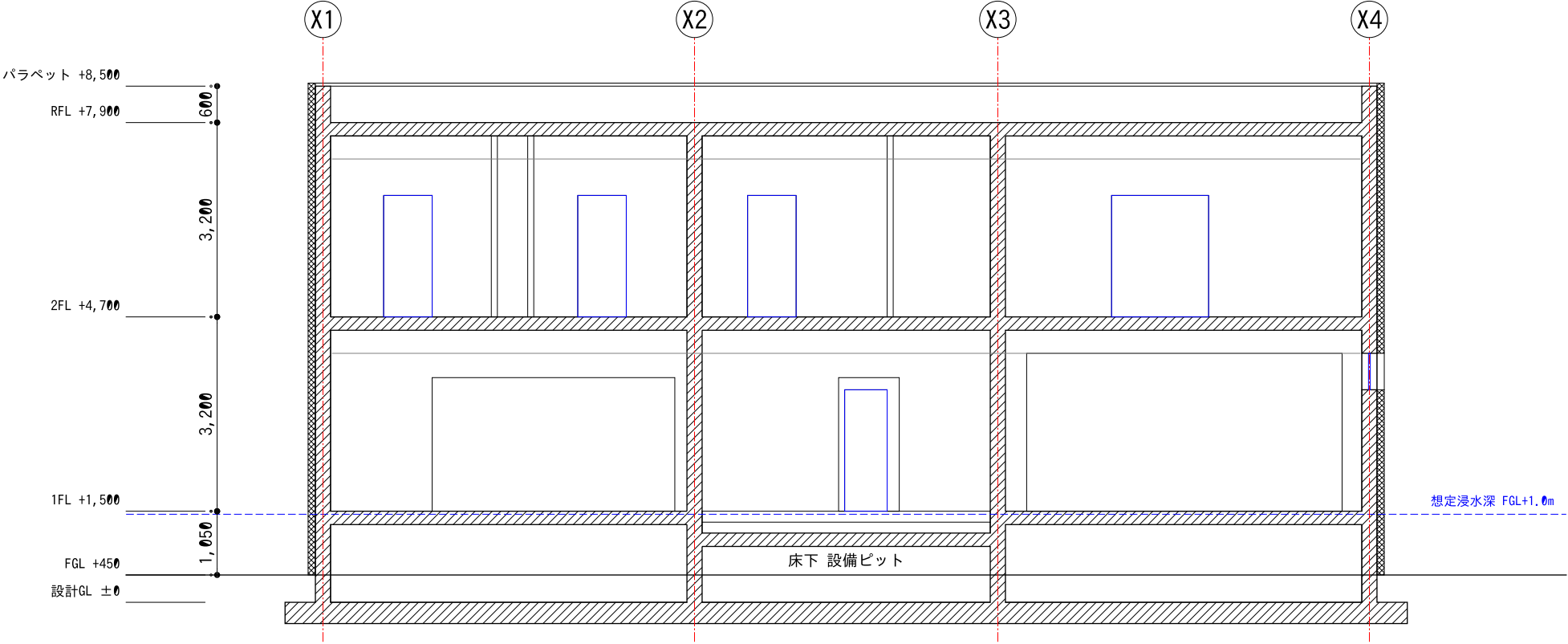
断面図 B-B（Y1-Y2間、LDK・玄関土間・ジム搬入扉を通る東西断面）
