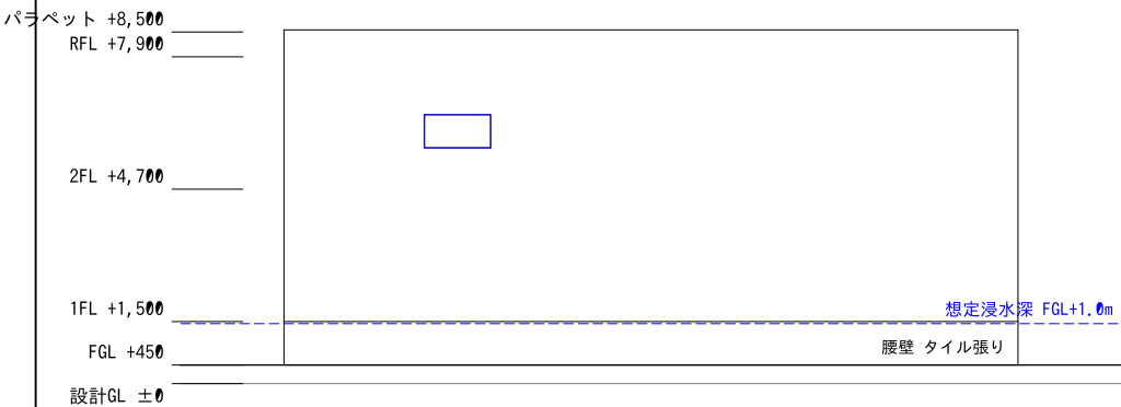
北立面図
