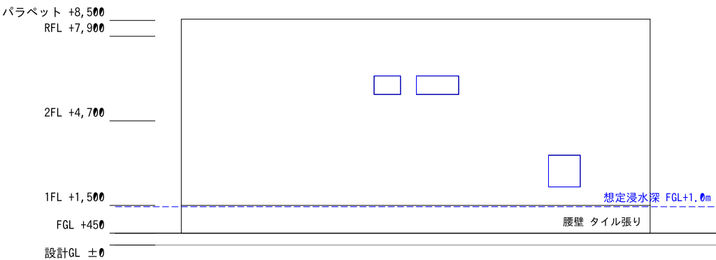
西立面図
