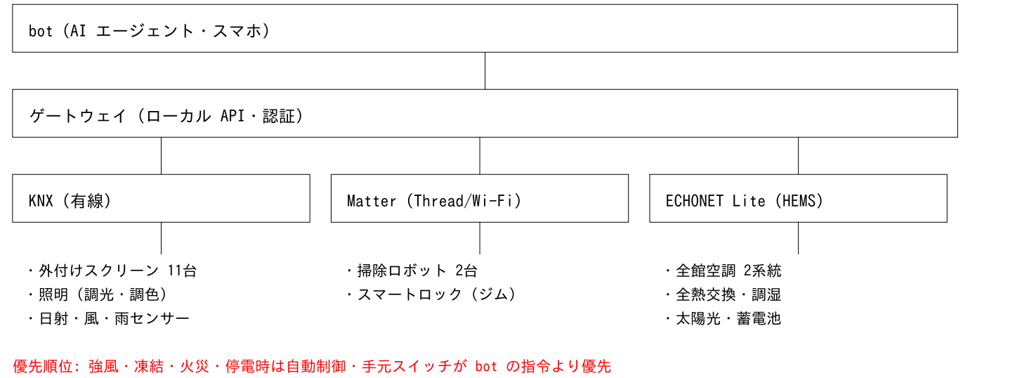
(1) 制御の構成
