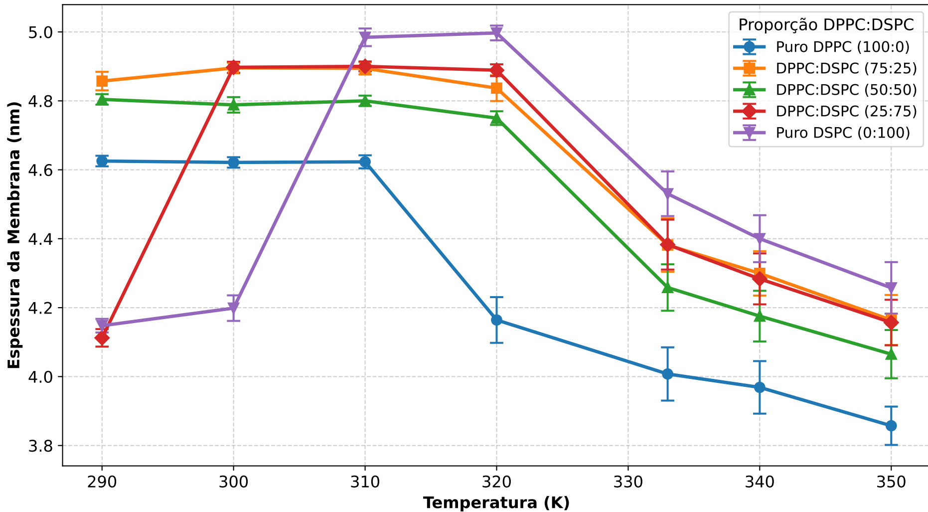
Perfil Termotrópico da Espessura da Bicamada (45W_L)
