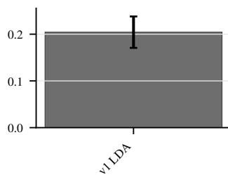
ECE
