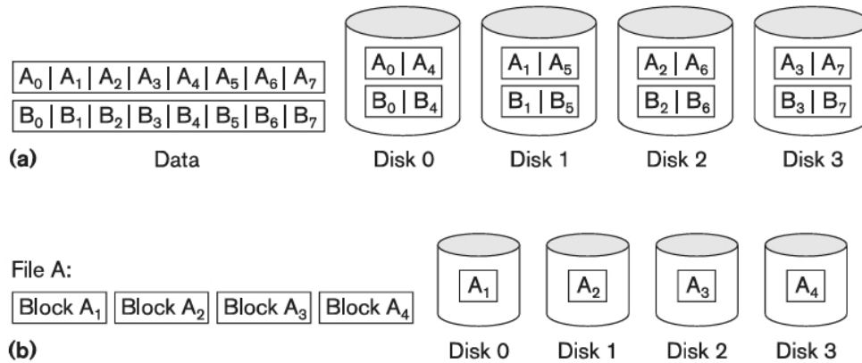
Figura 1: Comparação entre bit-level striping (a) e block-level striping (b) em um array de 4 discos. Em (a), bits sucessivos são distribuídos ciclicamente pelos discos; em (b), blocos inteiros são distribuídos em padrão round-robin . Adaptado de [2].
