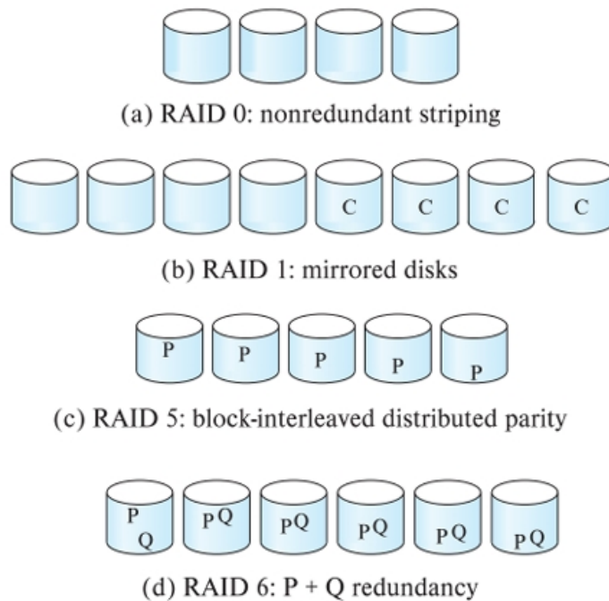
Figura 2: Visão geral das arquiteturas dos principais níveis RAID: (a) RAID 0 — striping sem redundância; (b) RAID 1 — espelhamento completo (C = cópia); (c) RAID 5 — paridade distribuída entre todos os discos (P); (d) RAID 6 — dupla paridade distribuída (P e Q). Adaptado de [2].
