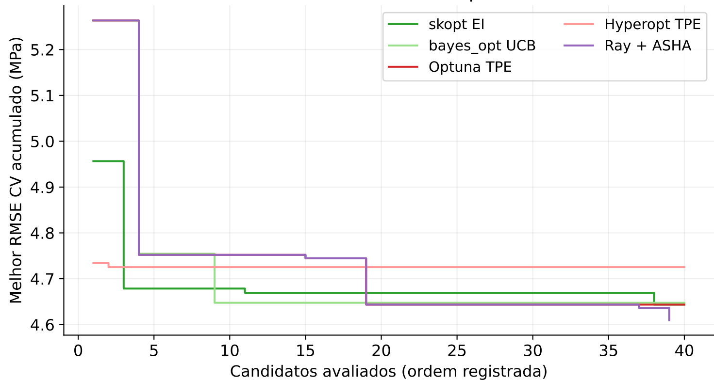
Bibliotecas: melhor RMSE CV completo acumulado
