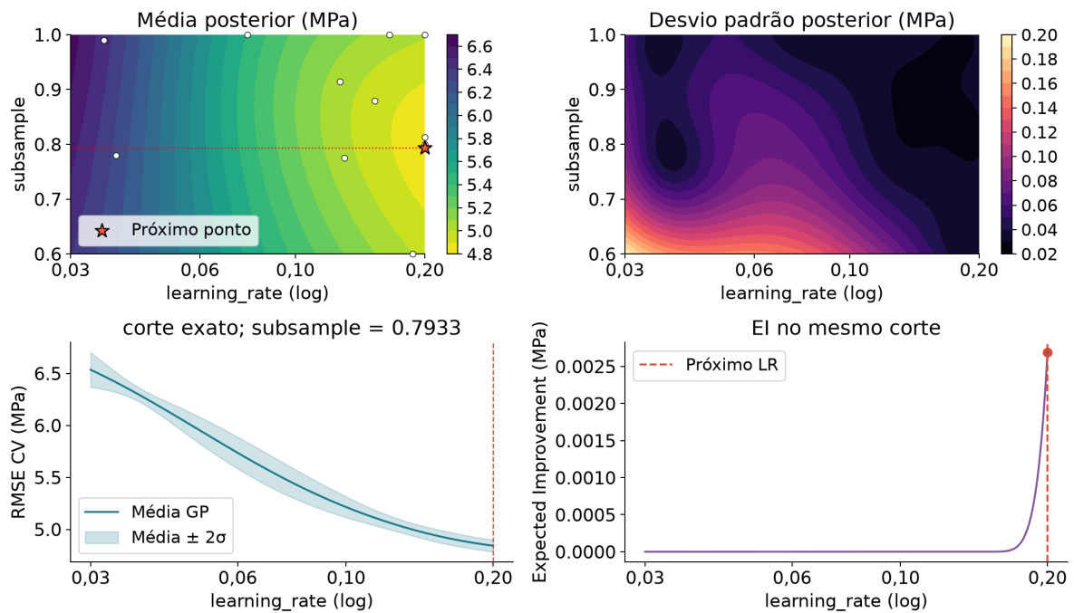
Figura 24. Posterior e EI antes da aquisição 7, com 11 observações. Candidato: \eta=0,2000 , s=0,7933 . As observações reais são exibidas no mapa 2D; o corte mantém o subsample fixo e não projeta pontos de outras seções.
