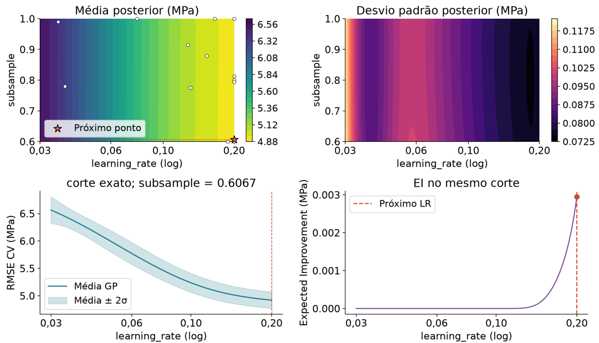
Figura 26. Posterior e EI antes da aquisição 9, com 13 observações. Candidato: \eta=0,2000 , s=0,6067 . As observações reais são exibidas no mapa 2D; o corte mantém o subsample fixo e não projeta pontos de outras seções.
