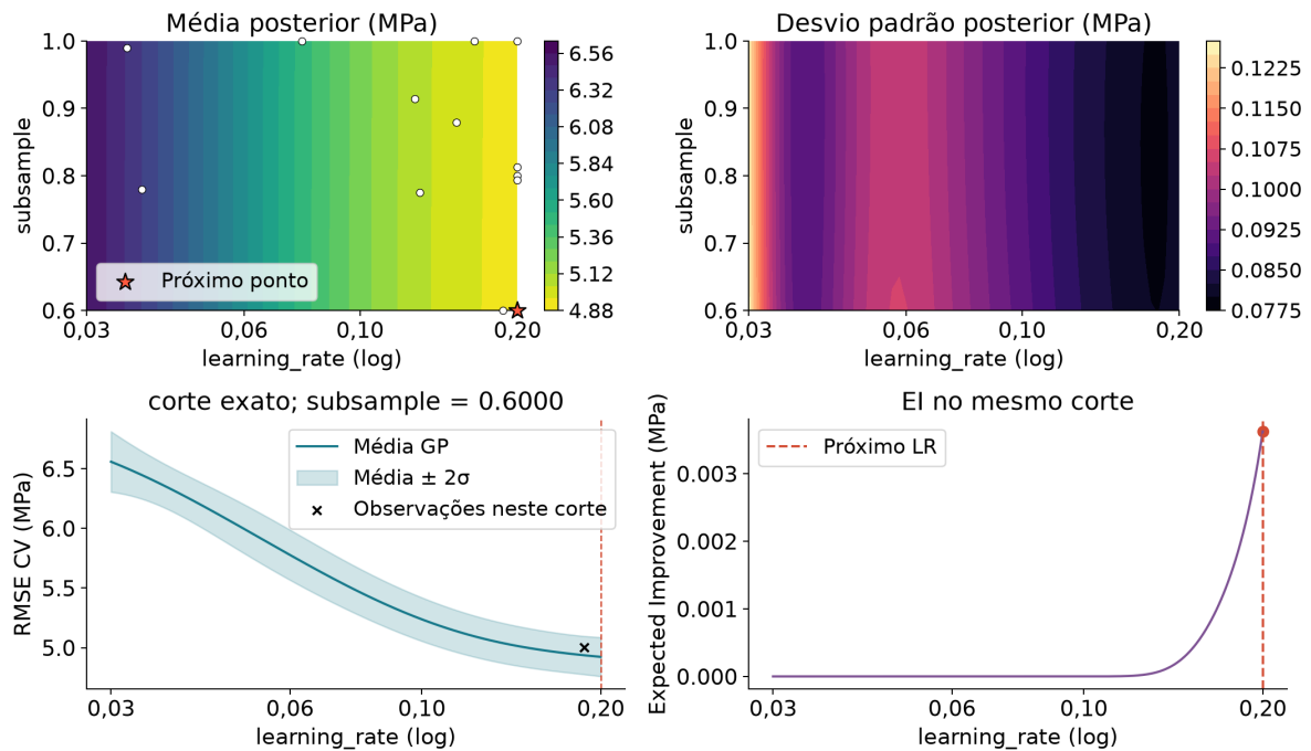
Figura 25. Posterior e EI antes da aquisição 8, com 12 observações. Candidato: \eta=0,2000 , s=0,6000 . As observações reais são exibidas no mapa 2D; o corte mantém o subsample fixo e não projeta pontos de outras seções.
