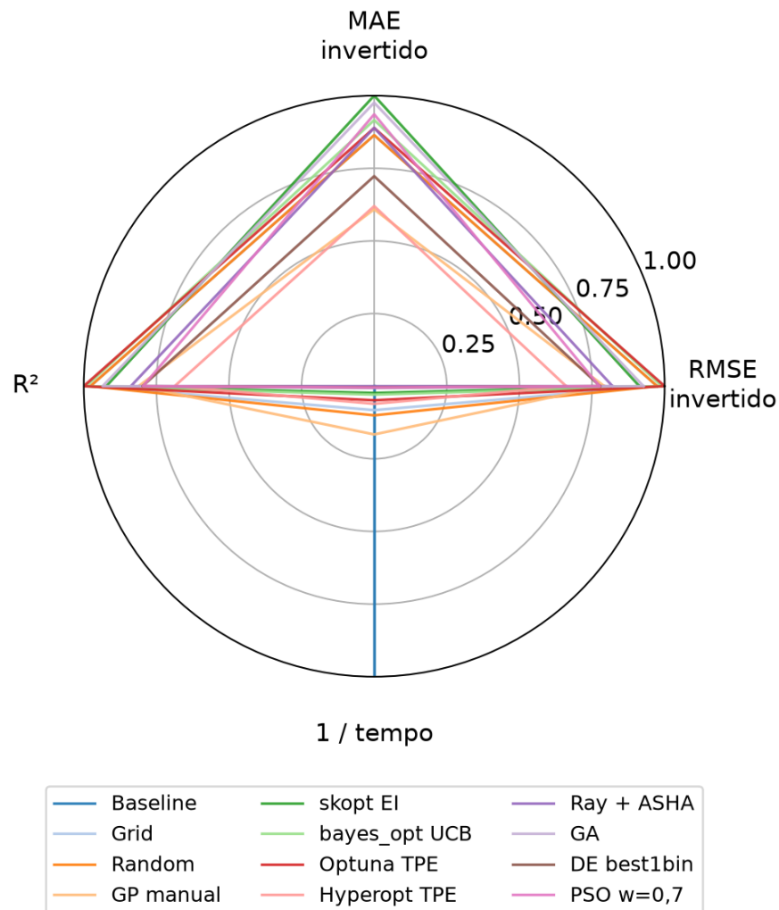
Figura 12. Radar dos 12 métodos principais: maior é melhor em todos os eixos; os limites são os do conjunto exibido.
