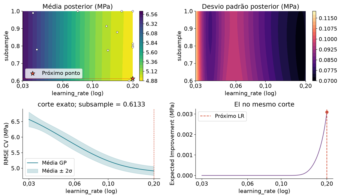
Figura 27. Posterior e EI antes da aquisição 10, com 14 observações. Candidato: \eta=0,2000 , s=0,6133 . As observações reais são exibidas no mapa 2D; o corte mantém o subsample fixo e não projeta pontos de outras seções.
