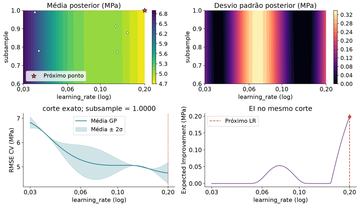
Figura 18. Posterior e EI antes da aquisição 1, com 5 observações. Candidato: \eta=0,2000 , s=1,0000 . As observações reais são exibidas no mapa 2D; o corte mantém o subsample fixo e não projeta pontos de outras seções.
