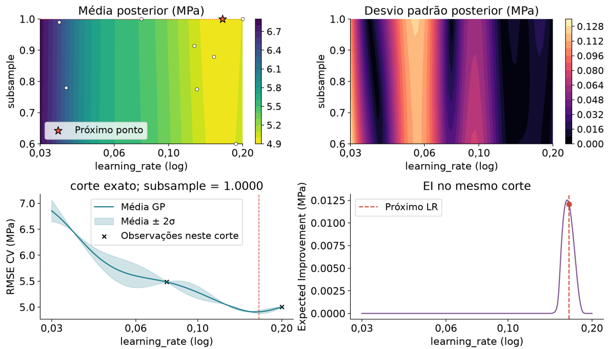
Figura 21. Posterior e EI antes da aquisição 4, com 8 observações. Candidato: \eta=0,1654 , s=1,0000 . As observações reais são exibidas no mapa 2D; o corte mantém o subsample fixo e não projeta pontos de outras seções.
