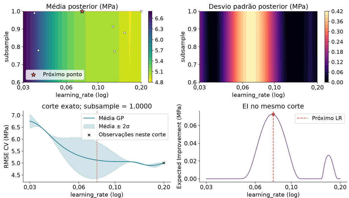
Figura 19. Posterior e EI antes da aquisição 2, com 6 observações. Candidato: \eta=0,0775 , s=1,0000 . As observações reais são exibidas no mapa 2D; o corte mantém o subsample fixo e não projeta pontos de outras seções.
