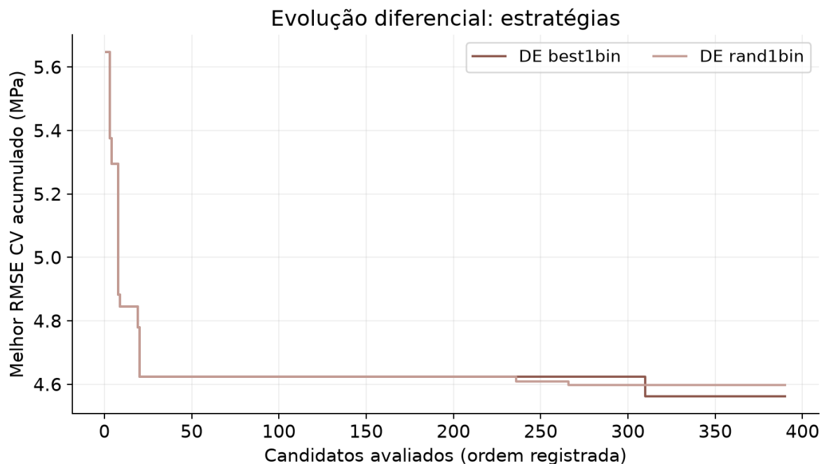
Figura 10. DE: melhor RMSE CV acumulado em best1bin e rand1bin.
