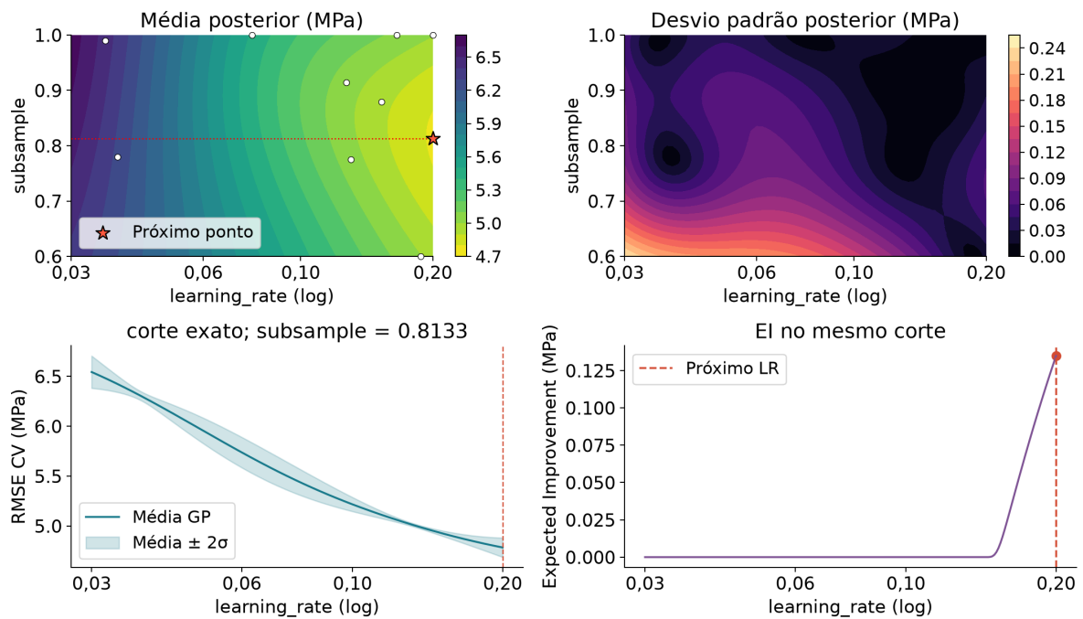
Figura 22. Posterior e EI antes da aquisição 5, com 9 observações. Candidato: \eta=0,2000 , s=0,8133 . As observações reais são exibidas no mapa 2D; o corte mantém o subsample fixo e não projeta pontos de outras seções.
