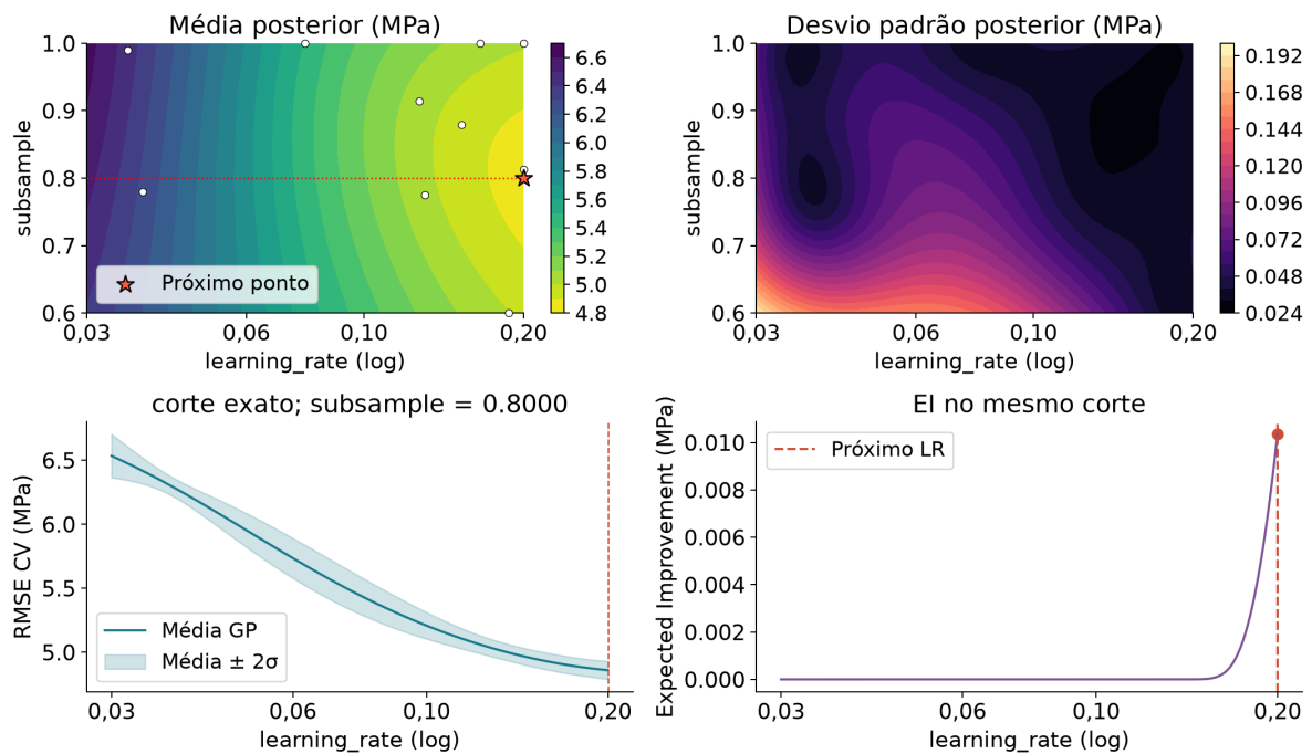
Figura 23. Posterior e EI antes da aquisição 6, com 10 observações. Candidato: \eta=0,2000 , s=0,8000 . As observações reais são exibidas no mapa 2D; o corte mantém o subsample fixo e não projeta pontos de outras seções.
