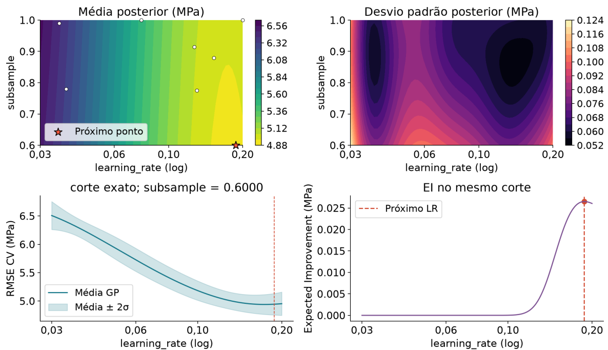
Figura 20. Posterior e EI antes da aquisição 3, com 7 observações. Candidato: \eta=0,1877 , s=0,6000 . As observações reais são exibidas no mapa 2D; o corte mantém o subsample fixo e não projeta pontos de outras seções.
