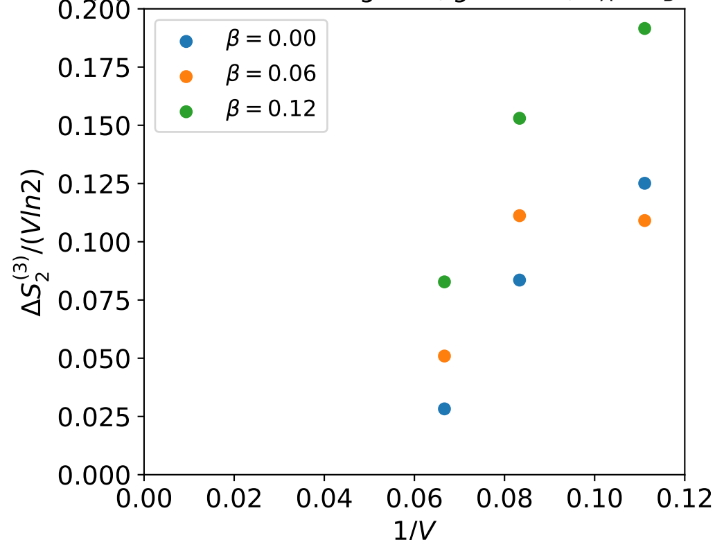
(d) Finite-size convergence, g = h = 1 , V_A = V_B = V_C
