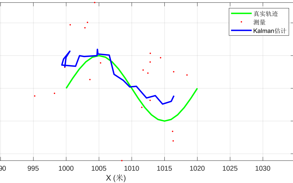
轨迹跟踪
