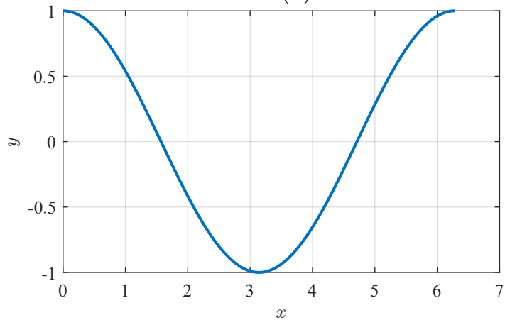
\cos(x)
