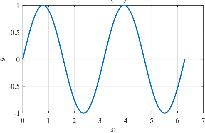
\sin(2x)
