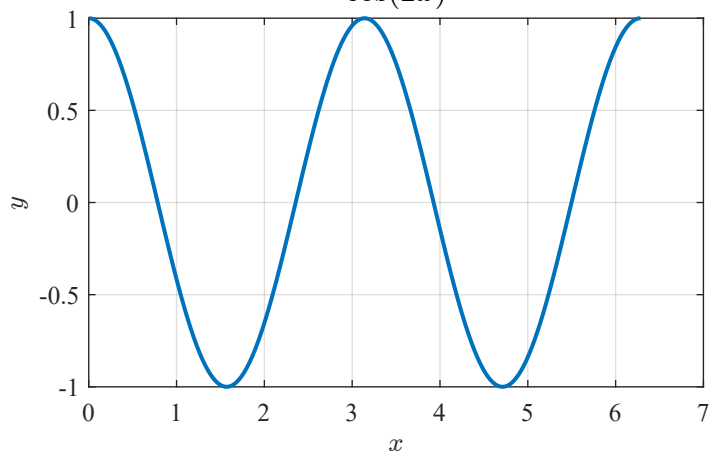
\cos(2x)
