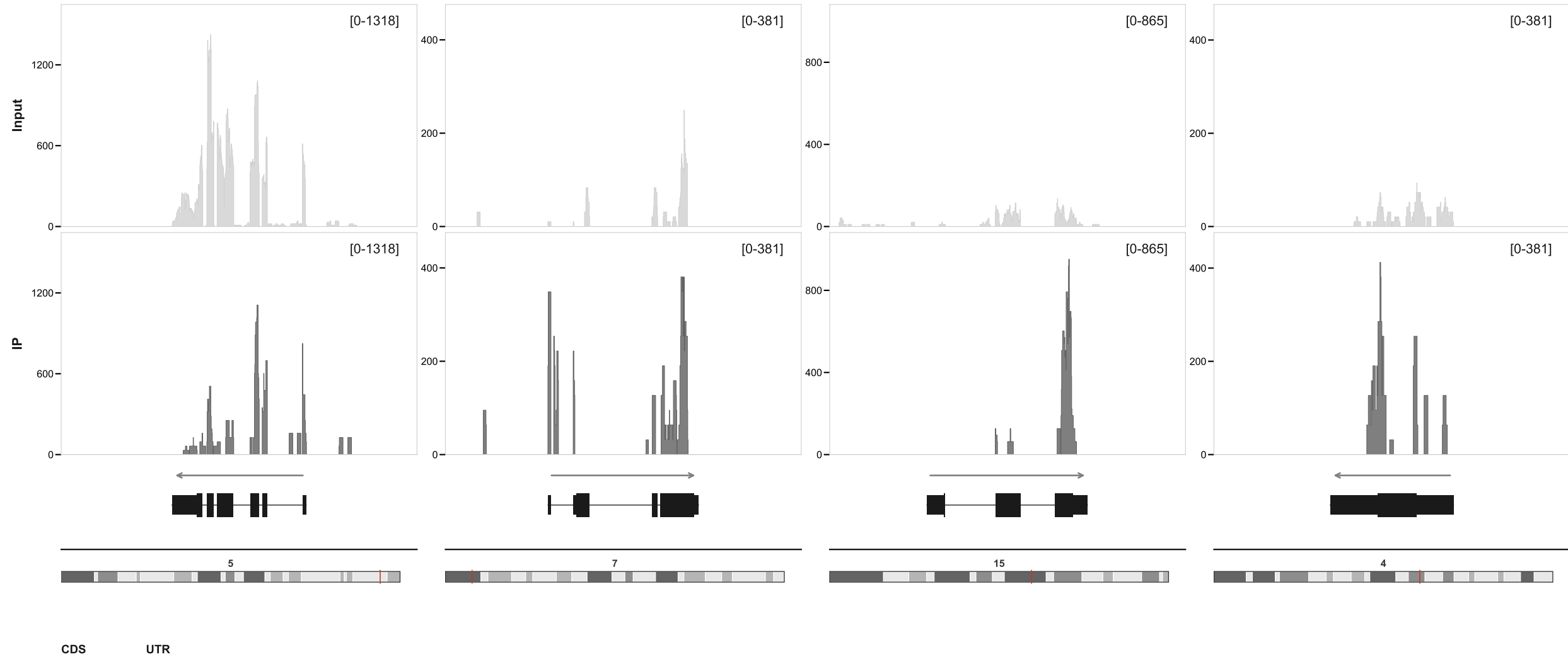
Actb | chr5:142,900,115-142,909,754
