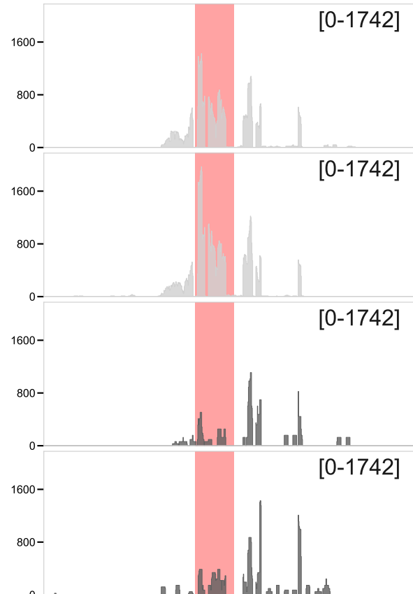
Actb | chr5:142,900,115-142,909,754
