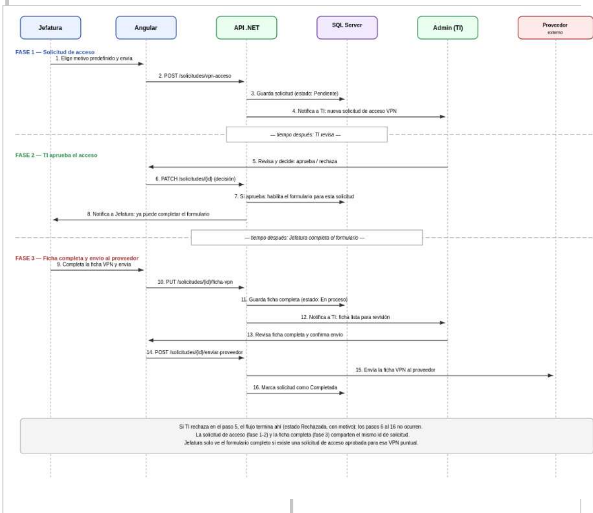
Figura 14. Diagrama de secuencia — Solicitud de VPN. Participan Jefatura, Angular, la API .NET, SQL Server, Admin (TI) y el Proveedor externo.
