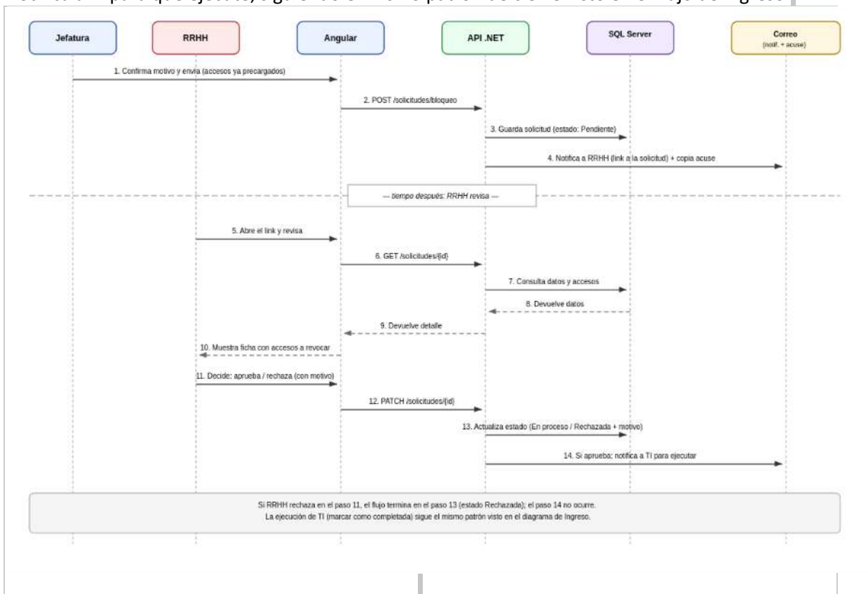
Figura 13. Diagrama de secuencia — Crear y revisar solicitud de Bloqueo. Participan Jefatura, RRHH, Angular, la API.NET, SQL Server y el correo de notificación.
