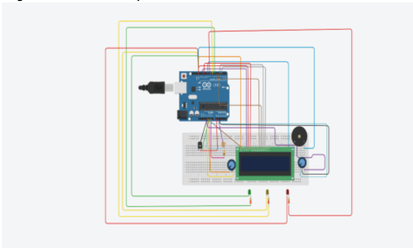
Figura 1 – Circuito Completo do Sistema
