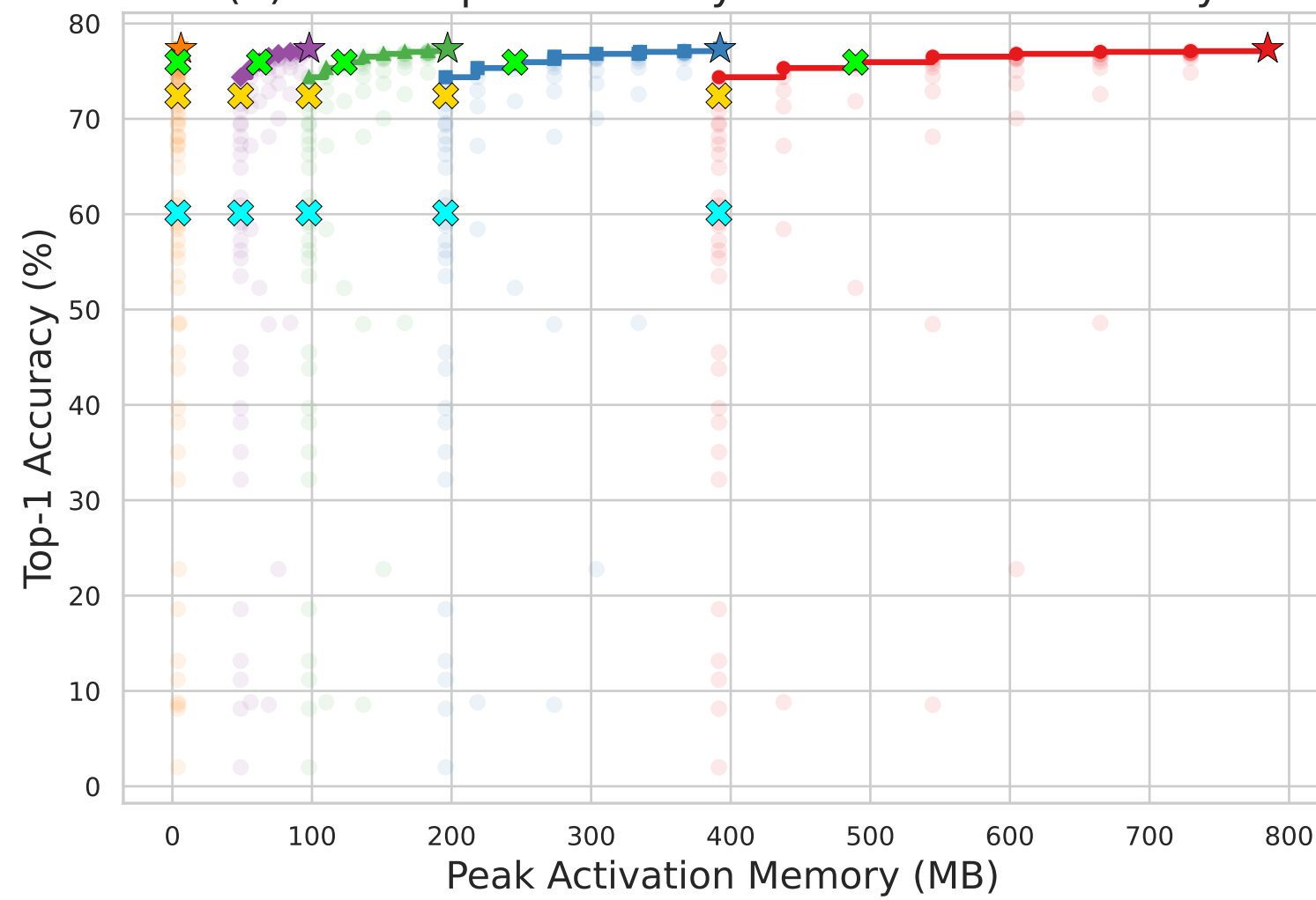
(d) GPU: Top-1 Accuracy vs. Activation Memory
