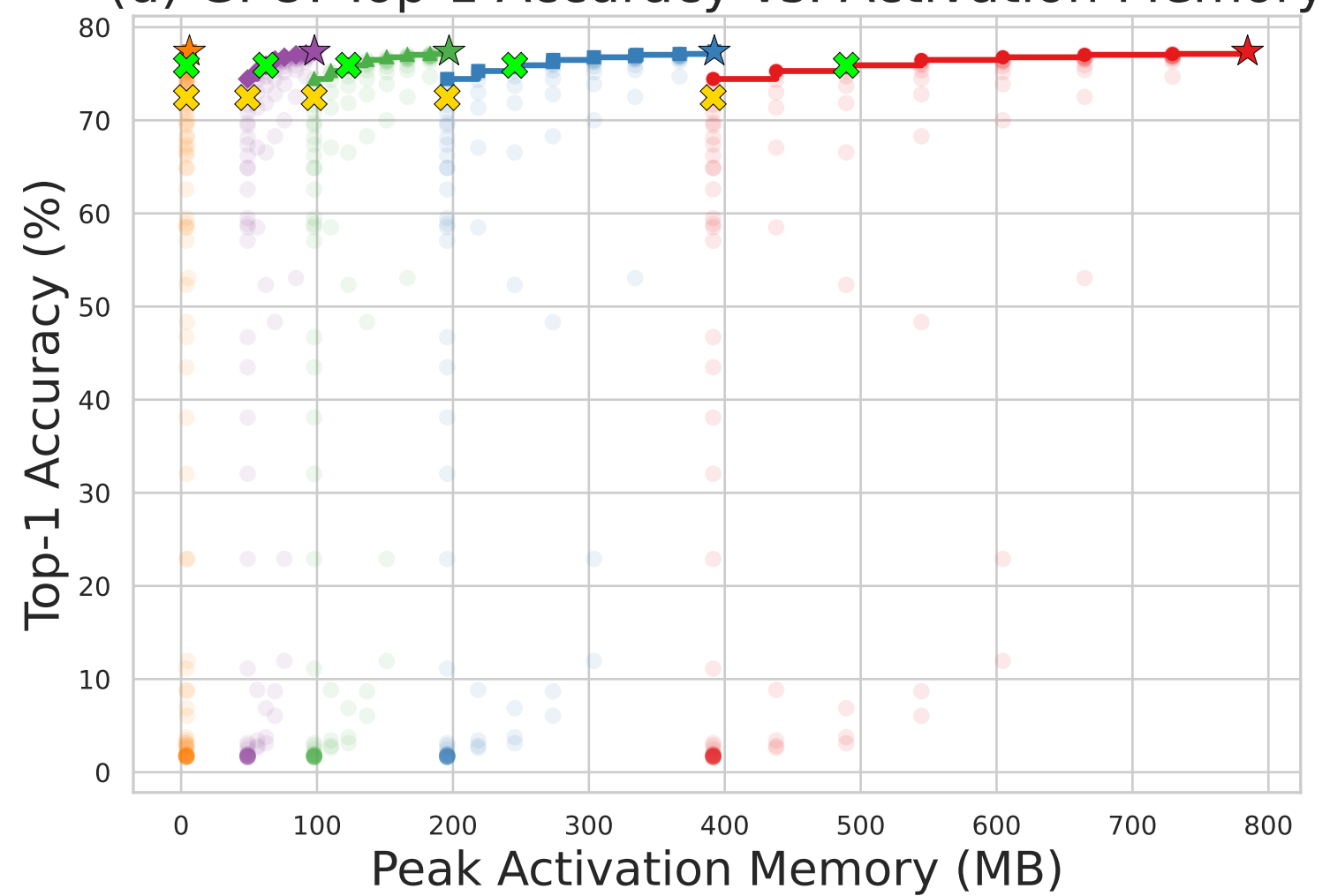
(d) GPU: Top-1 Accuracy vs. Activation Memory
