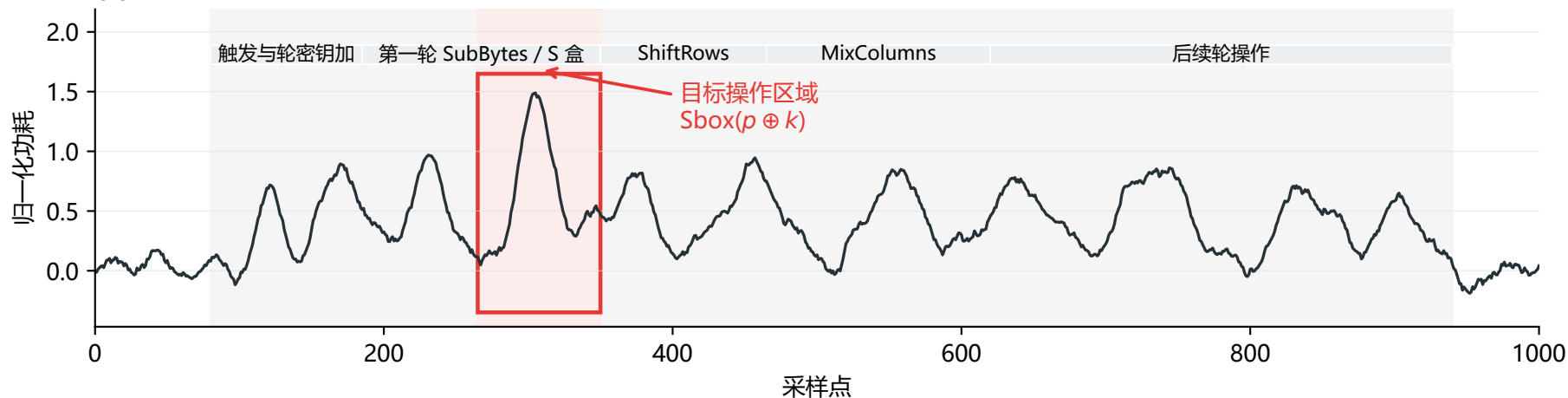
(a) 完整功耗曲线：从完整 AES 加密轨迹中定位目标 S 盒泄漏区域
