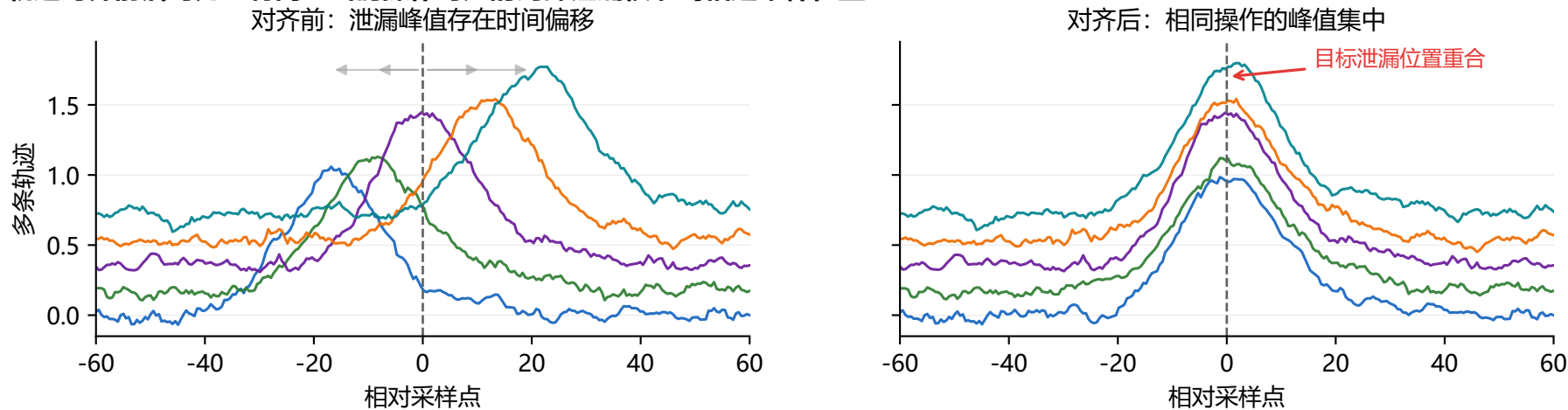
(c) 轨迹对齐前后对比：将同一密码操作对应的局部泄漏校准到相近采样位置
