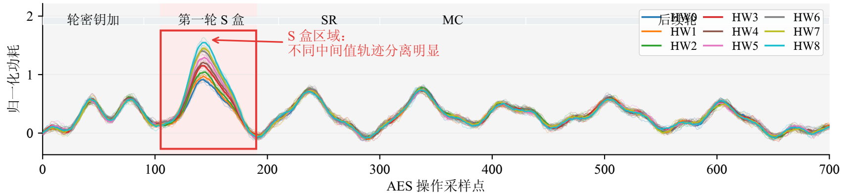
(a) AES 操作区间内多条功耗轨迹：S 盒区域类别区分更明显
