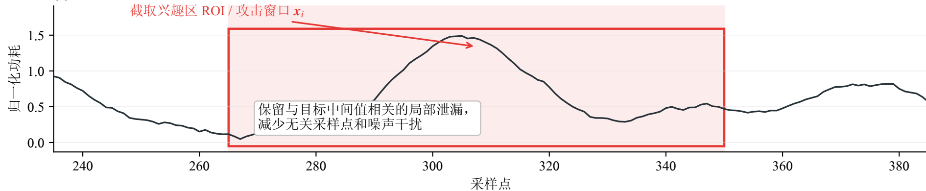
(b) 兴趣区截取：以第一轮 S 盒输出为目标截取局部攻击窗口
