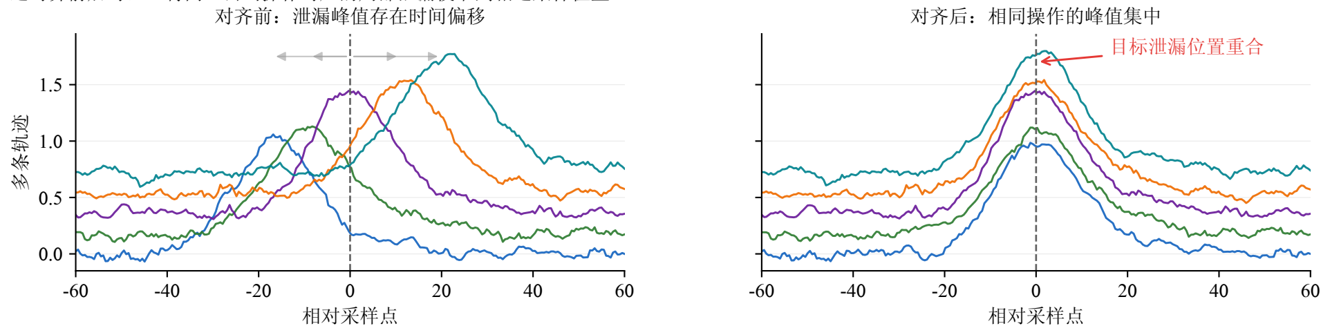
(c) 轨迹对齐前后对比：将同一密码操作对应的局部泄漏校准到相近采样位置
