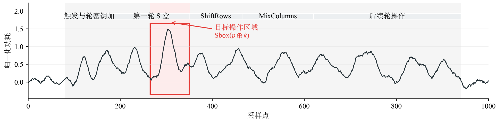
(a) 完整功耗曲线：从完整 AES 加密轨迹中定位目标 S 盒泄漏区域
