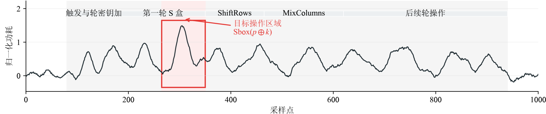
(a) 完整功耗曲线：从完整 AES 加密轨迹中定位目标 S 盒泄漏区域
