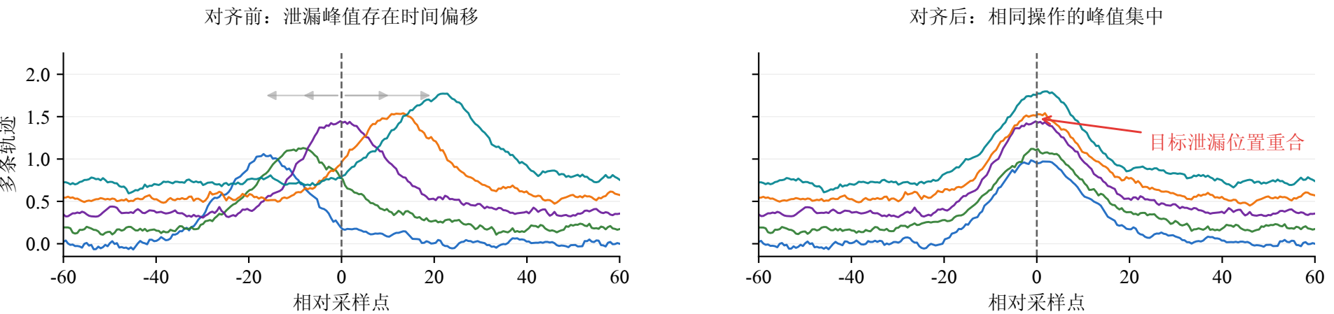
(c) 轨迹对齐前后对比：将同一密码操作对应的局部泄漏校准到相近采样位置
